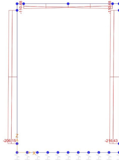
Sforzo normale
