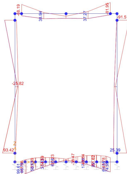
Momento Flettente
