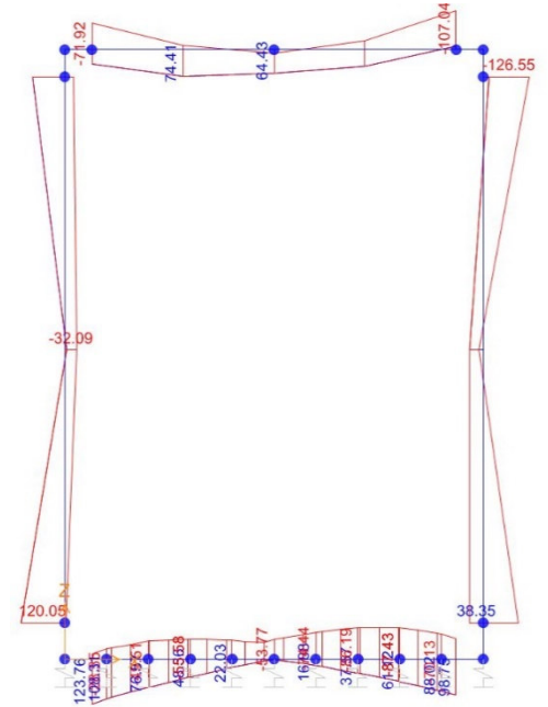
Momento Flettente
