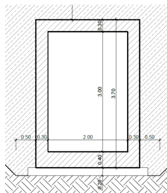
Figura 1c. Sezione trasversale dello scatolare
