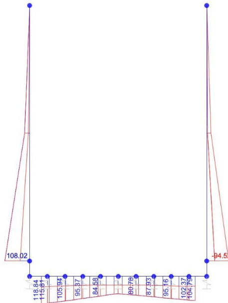
Momento Flettente
