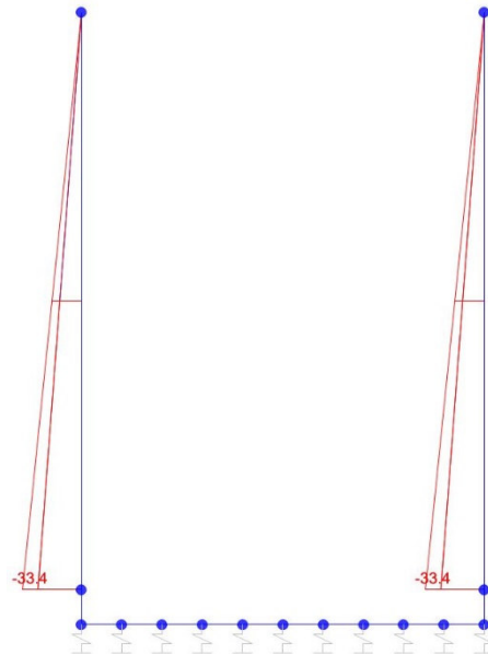
Sforzo normale
