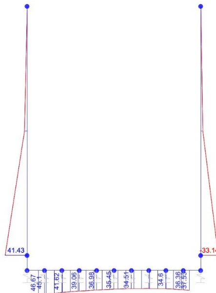
Momento flettente
