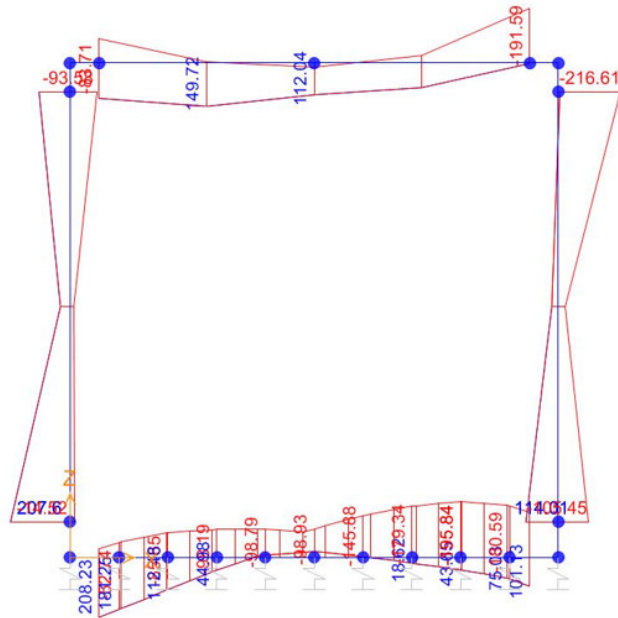
Momento Flettente
