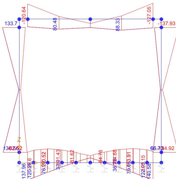
Momento Flettente
