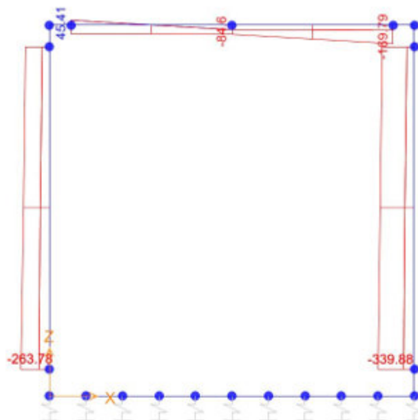
Sforzo normale
