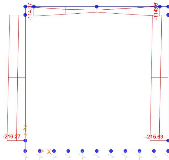
Sforzo normale
