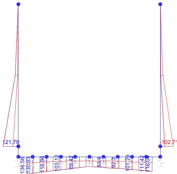
Momento Flettente
