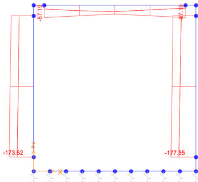
Sforzo normale
