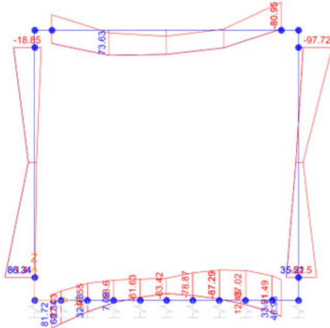
Momento Flettente
