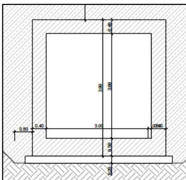
Figura 1c. Sezione trasversale dello scatolare
