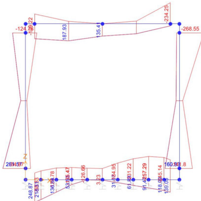
Momento Flettente
