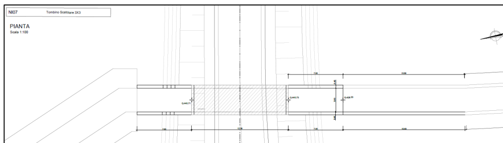
Figura 1a. Stralcio planimetrico dello scatolare
