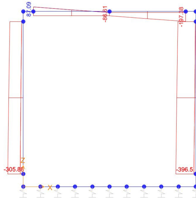
Sforzo normale
