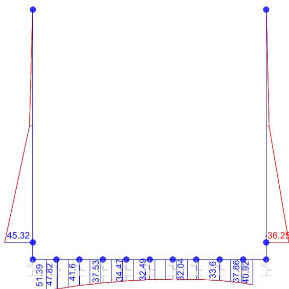
Momento flettente
