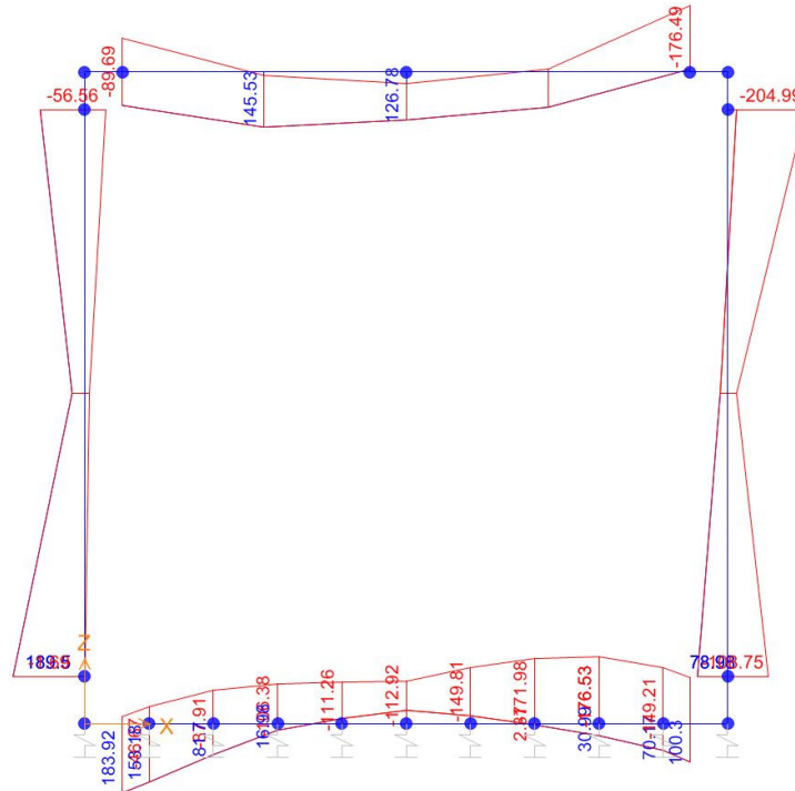
Momento Flettente
