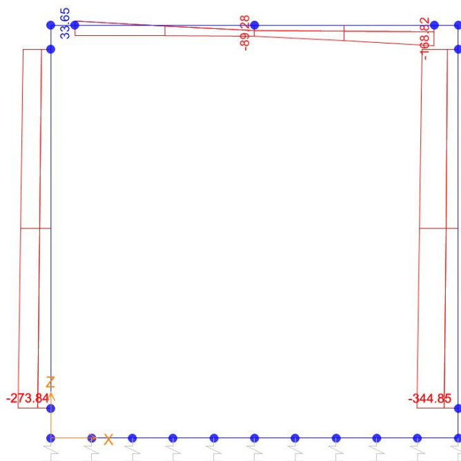
Sforzo normale
