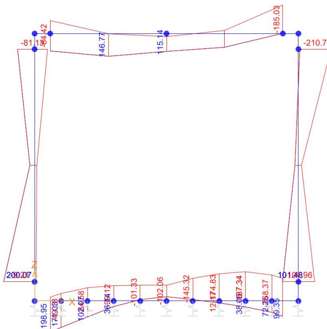
Momento Flettente
