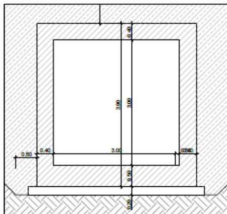
Figura 1c. Sezione trasversale dello scatolare
