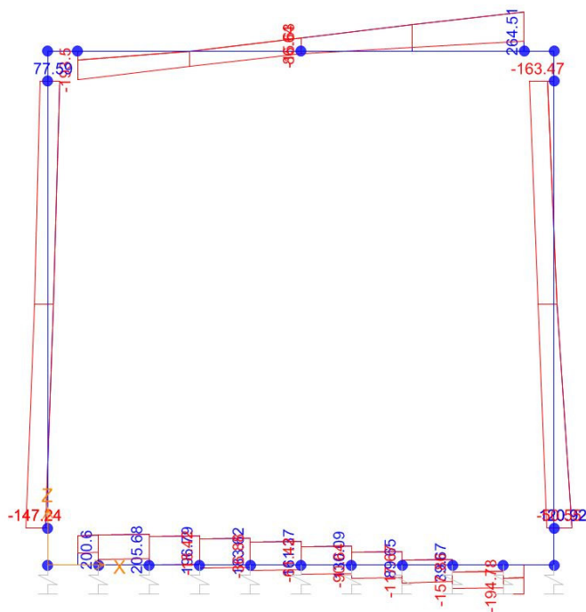
Taglio
