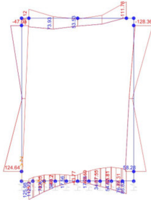
Momento Flettente
