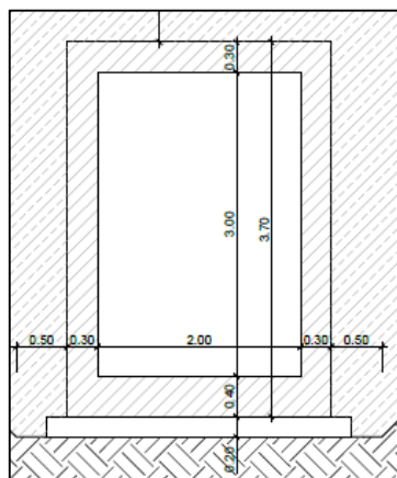
Figura 1c. Sezione trasversale dello scatolare
