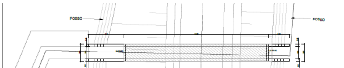
Figura 1a. Sezione planimetrica dello scatolare
