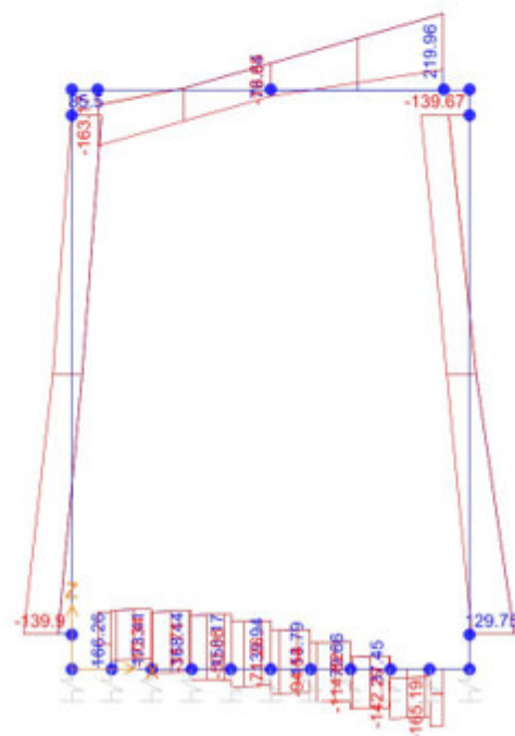
Taglio
