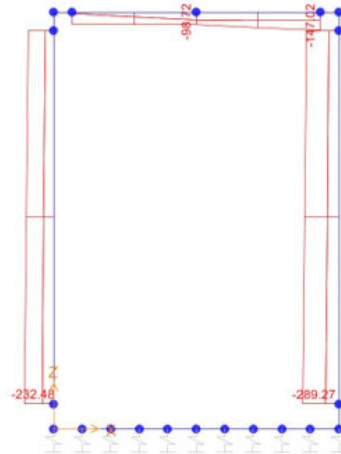
Sforzo normale
