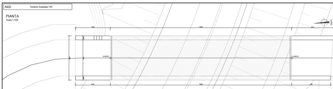
Figura 1a. Stralcio planimetrico dello scatolare
