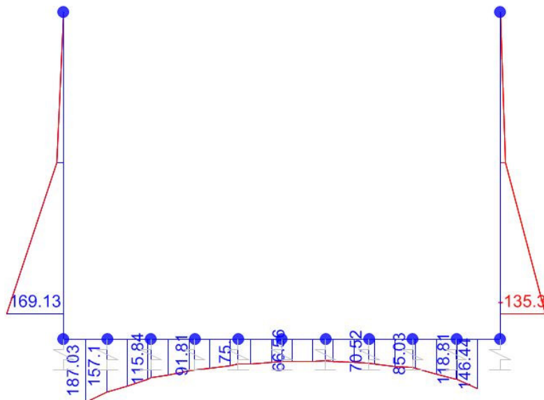
Momento flettente
