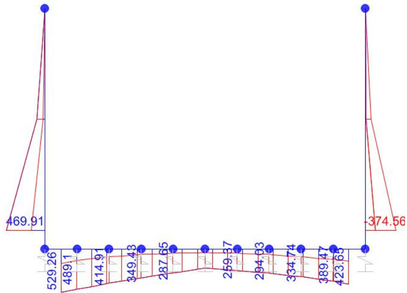
Momento Flettente
