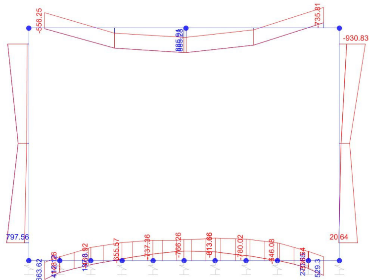
Momento Flettente
