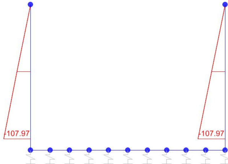
Sforzo normale
