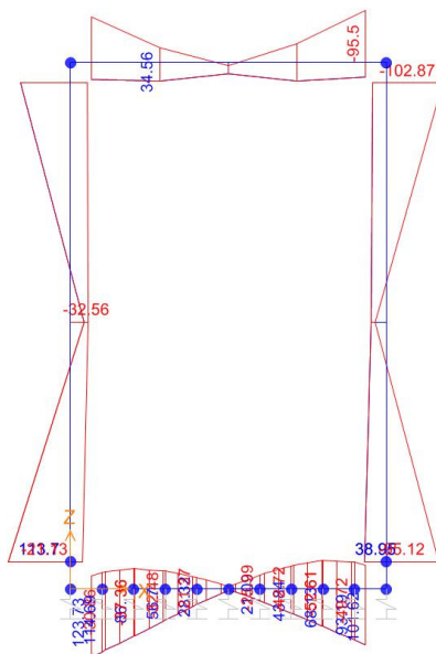
Momento Flettente
