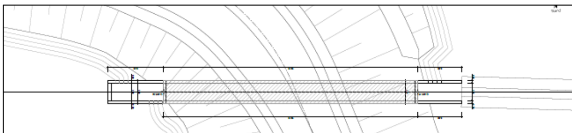
Figura 1a. Stralcio planimetrico dello scatolare
