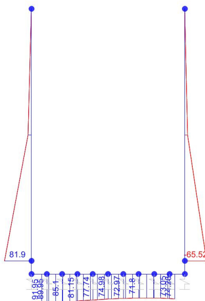
Momento flettente
