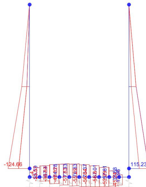
Taglio
