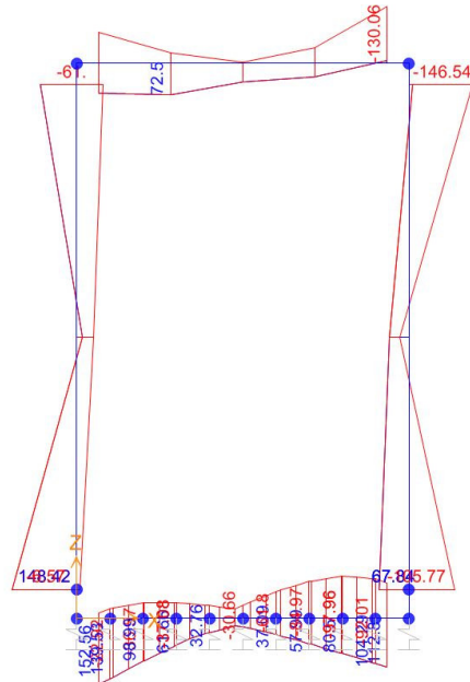
Momento Flettente
