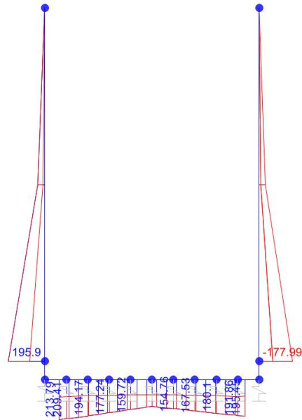
Momento Flettente
