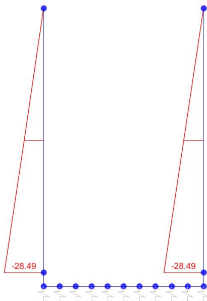
Sforzo normale
