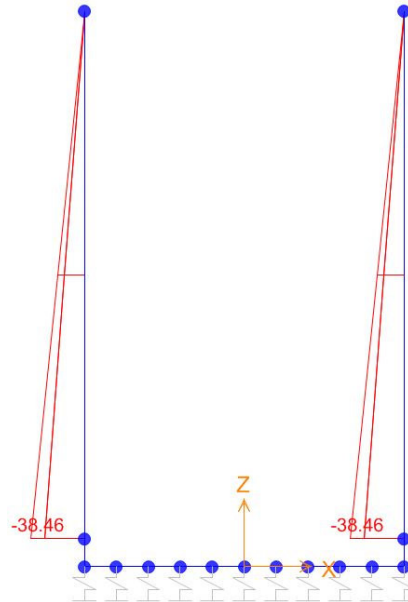
Sforzo normale
