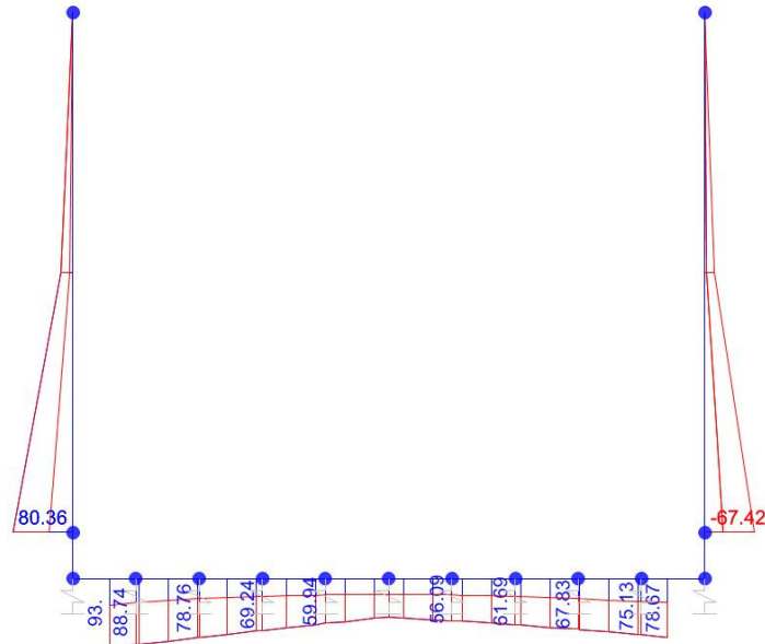
Momento Flettente
