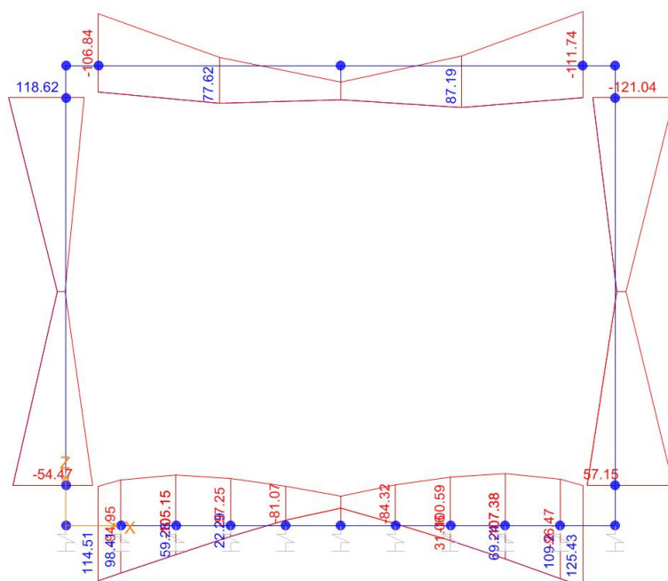
Momento Flettente
