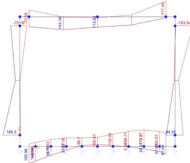
Momento Flettente
