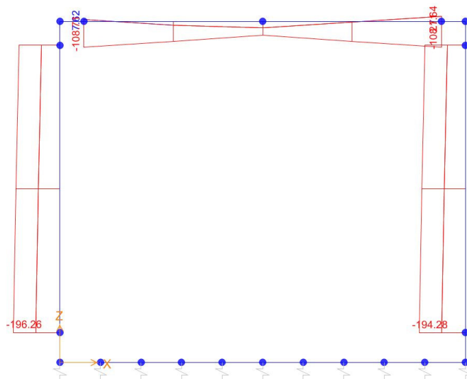
Sforzo normale
