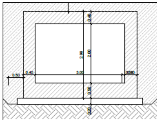
Figura 1c. Sezione trasversale dello scatolare
