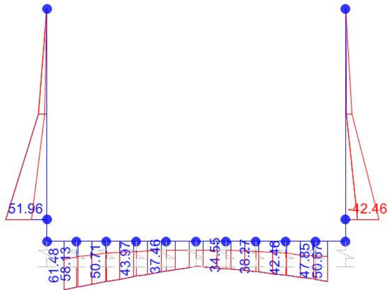
Momento Flettente
