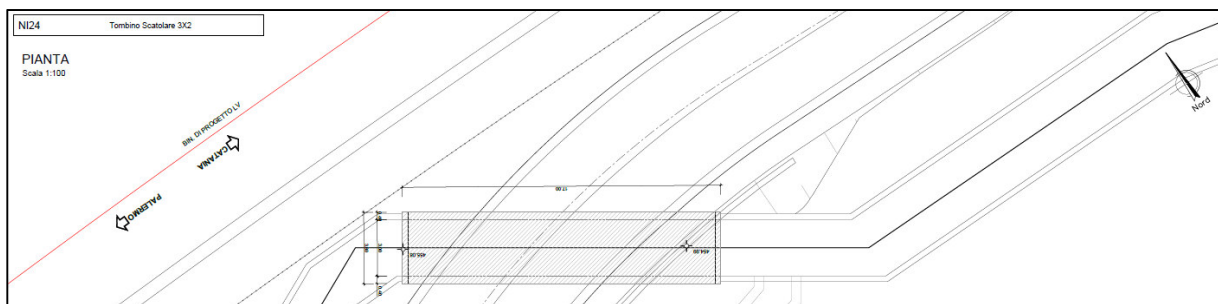
Figura 1a. Stralcio planimetrico dello scatolare
