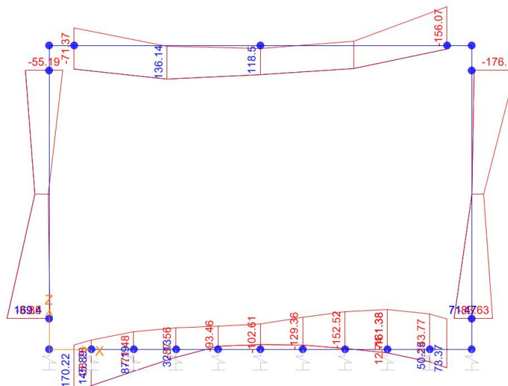
Momento Flettente
