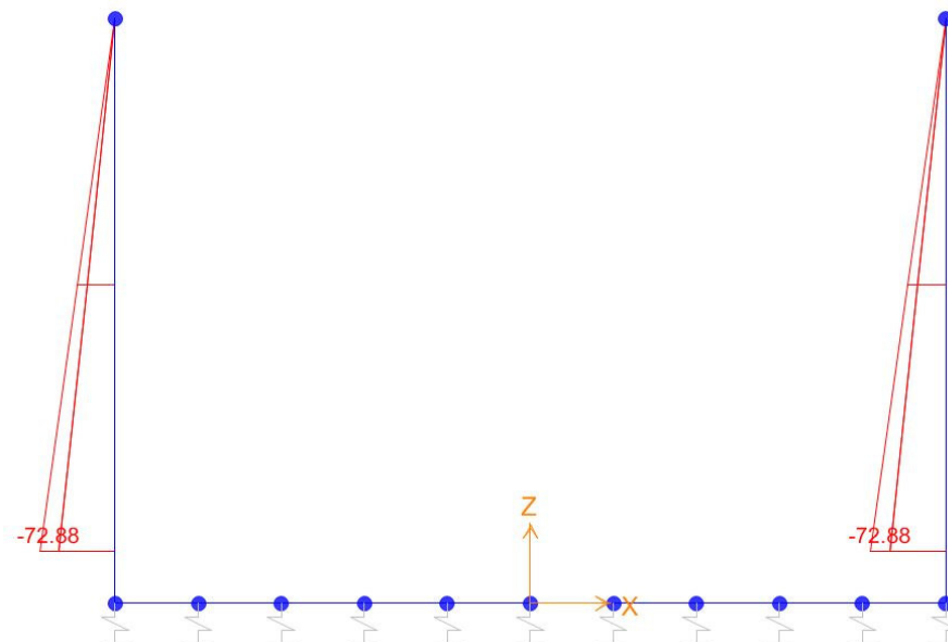
Sforzo normale
