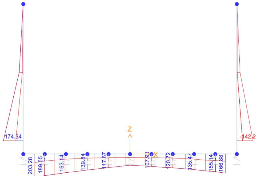
Momento Flettente
