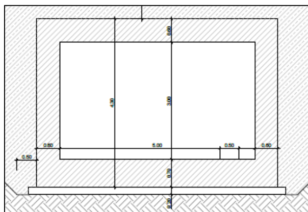
Figura 1c. Sezione trasversale dello scatolare
