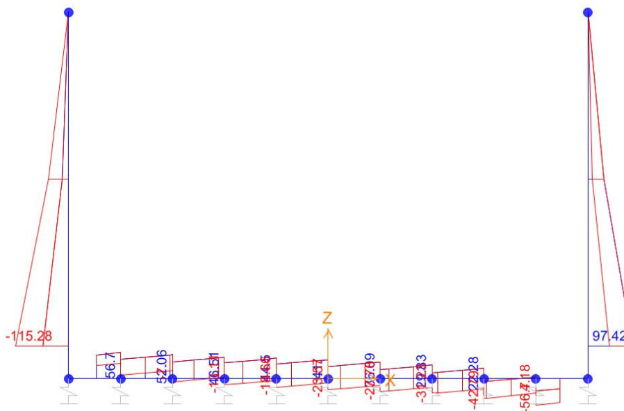
Taglio
