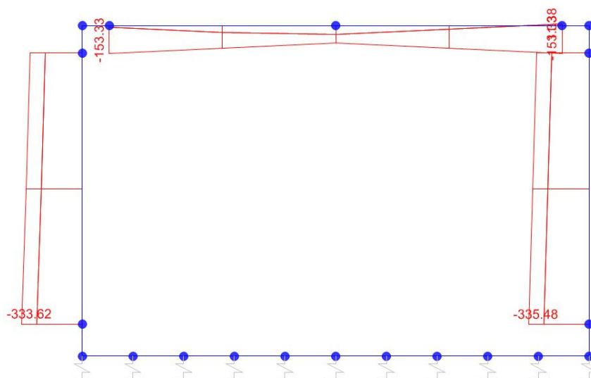
Sforzo normale
