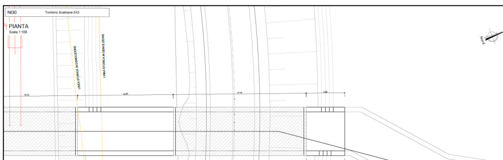
Figura 1a. Stralcio planimetrico dello scatolare
