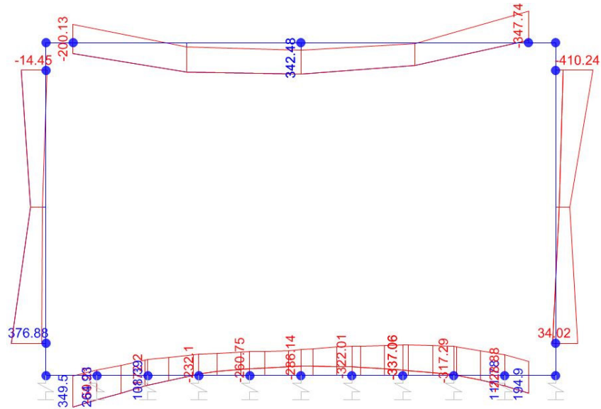
Momento Flettente
