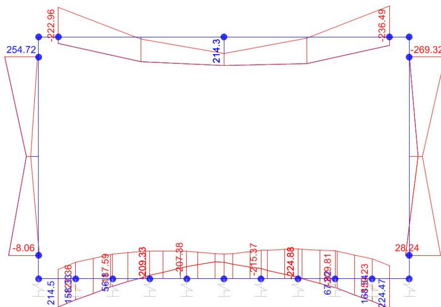
Momento Flettente
