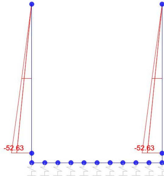
Sforzo normale
