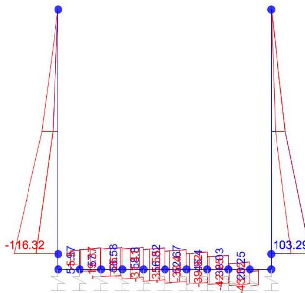
Taglio
