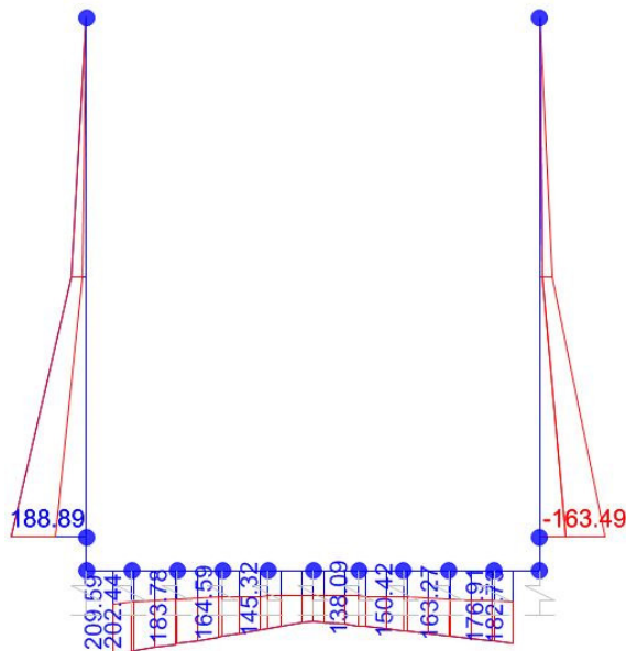
Momento Flettente
