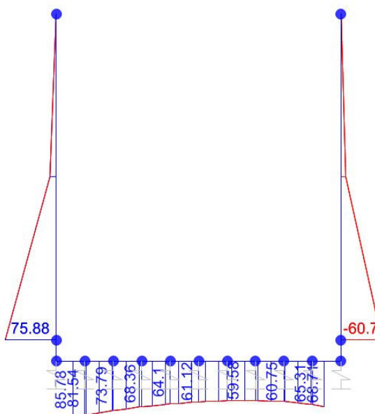
Momento flettente
