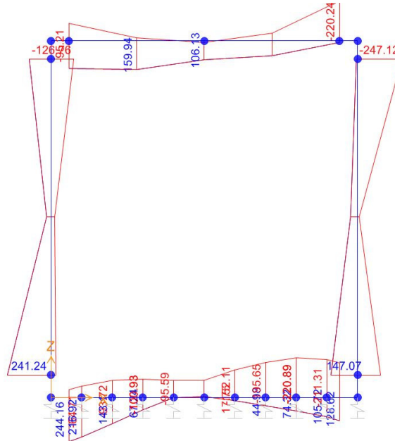
Momento Flettente
