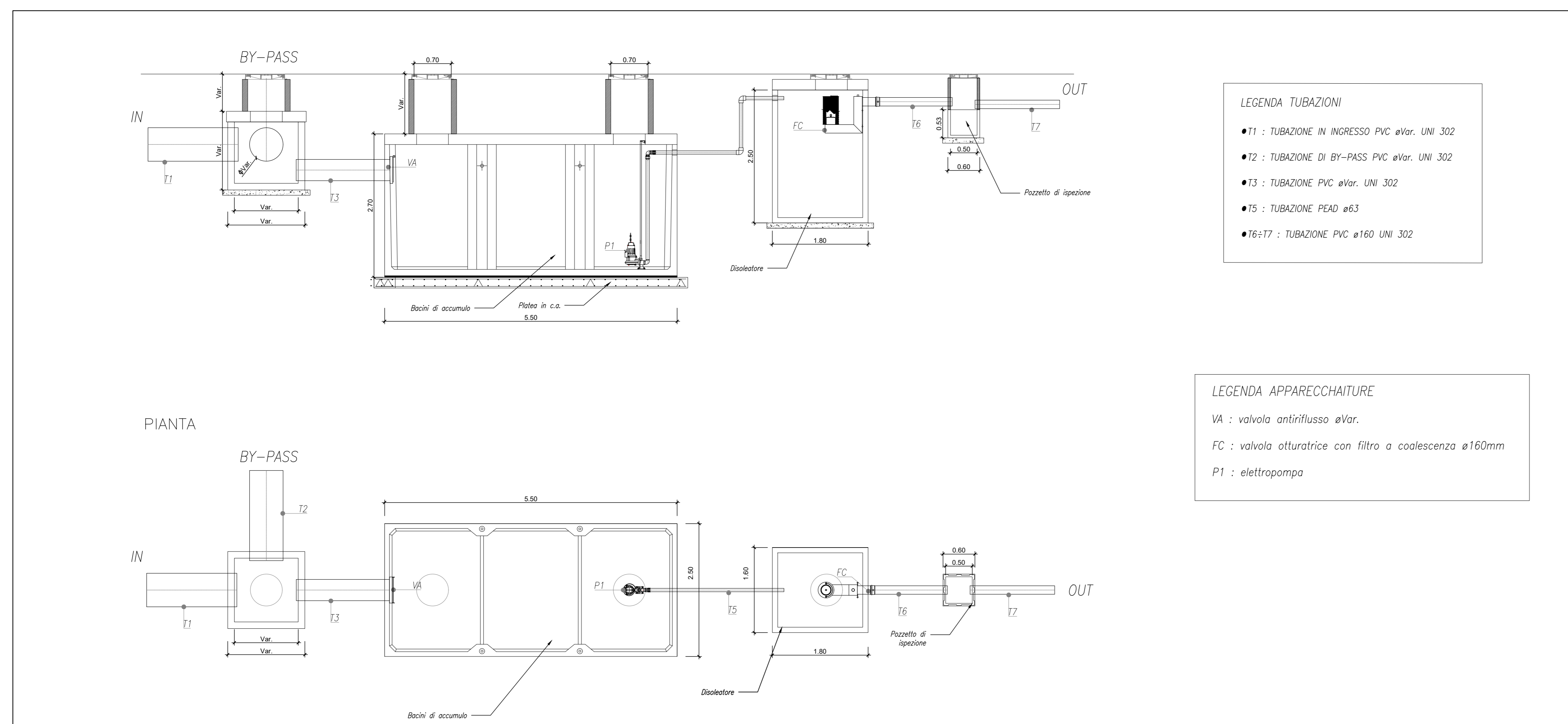
VASCA DI PRIMA PIOGGIA IN DISCONTINUO Scala 1:50
