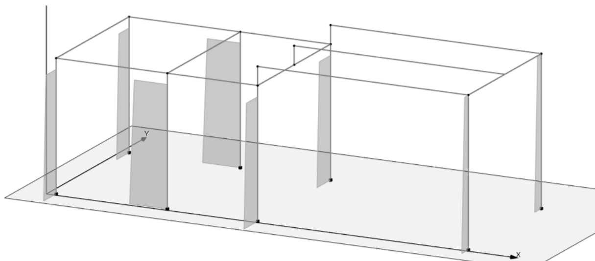
Figura 7.1-9 Diagramma dello sforzo assiale P – COMB_SLU_CC25.
