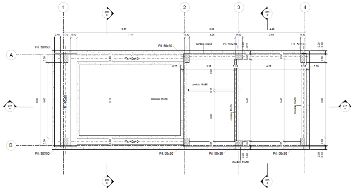
Carpenteria Fondazione 1 : 50
