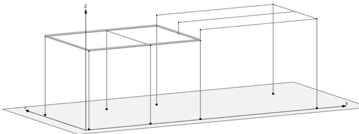
Figura 7.1-13 Schemi di carico - Tamponature
