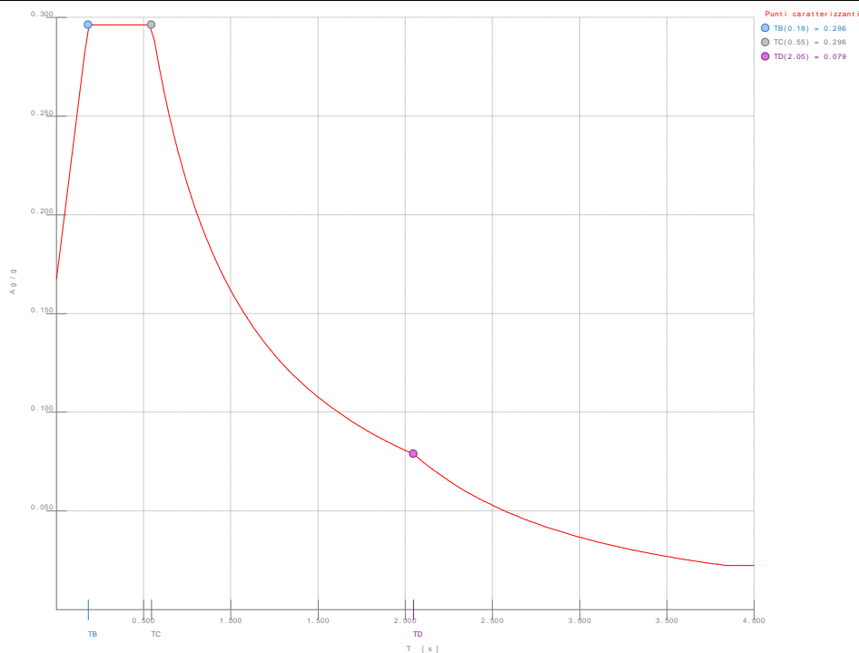
Spettro SND
