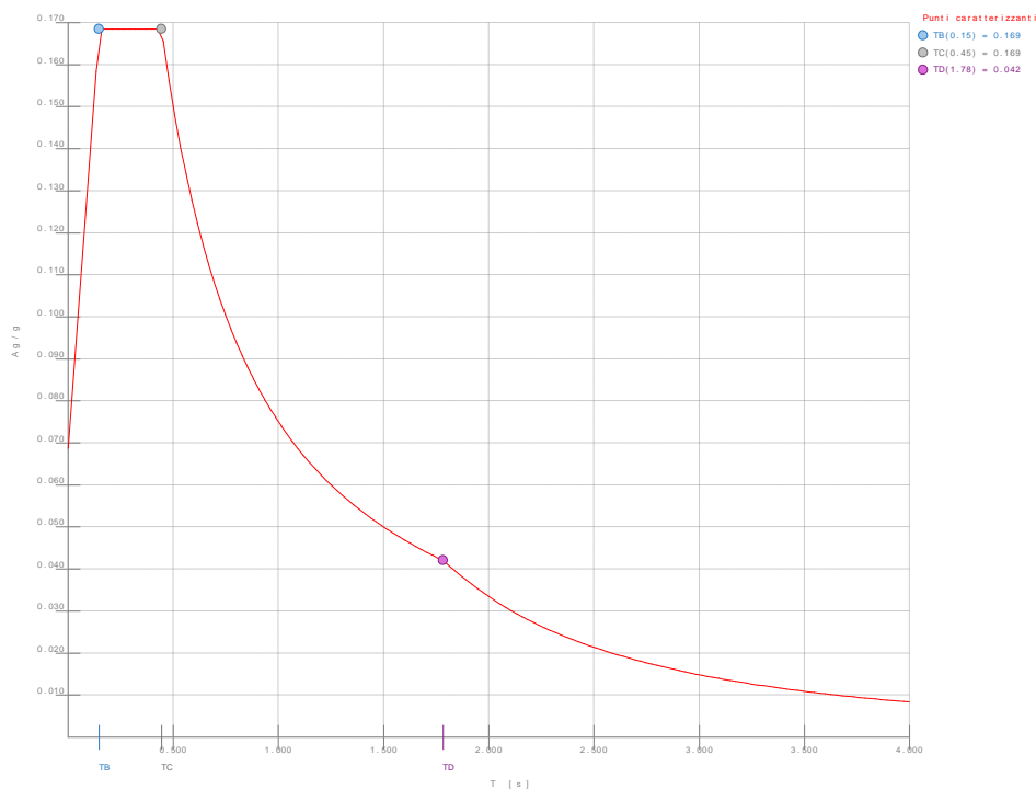
Spettro SLO
