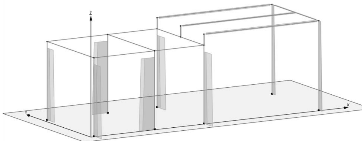
Figura 7.1-8 Diagramma dello sforzo assiale P – COMB_SLV_CC1.
