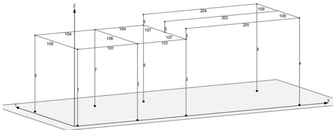
Figura 7.1-3 Numerazione aste.
