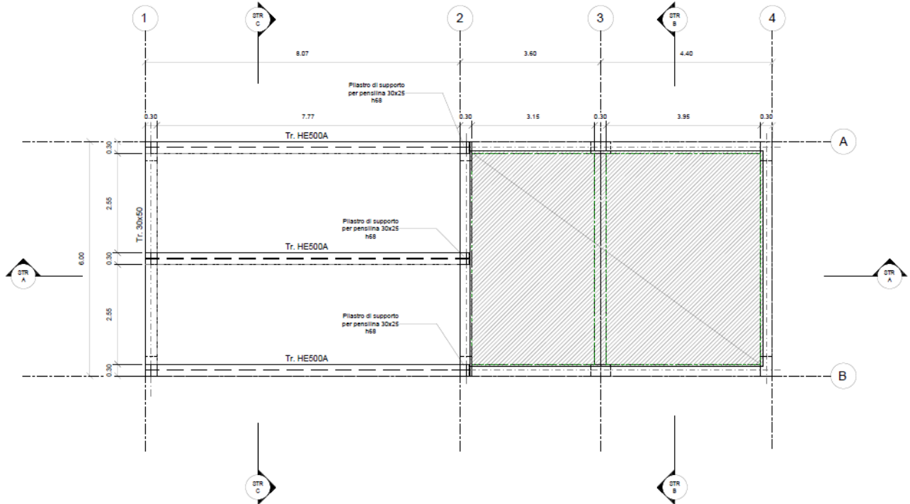
Carpenteria Parapetto 1 : 50
