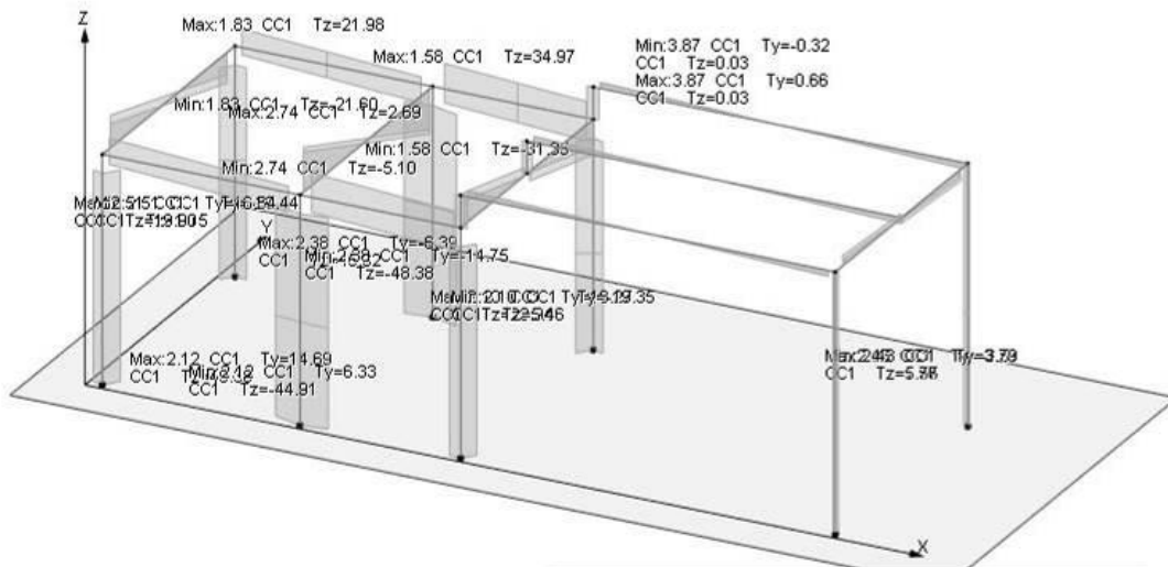
Figura 7.1-7 Diagramma del taglio V2 – COMB_INV_SLV_CC1.
