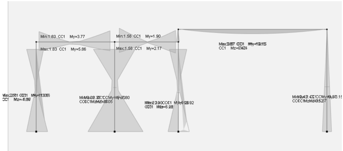
Figura 7.1-6 Diagramma dei momenti M3 – COMB_INV_SLV_CC1 – Telaio longitudinale.
