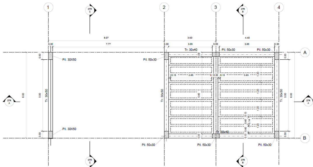
Carpenteria Copertura 1 : 50
