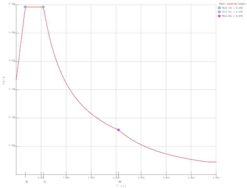
Spettro SLV
