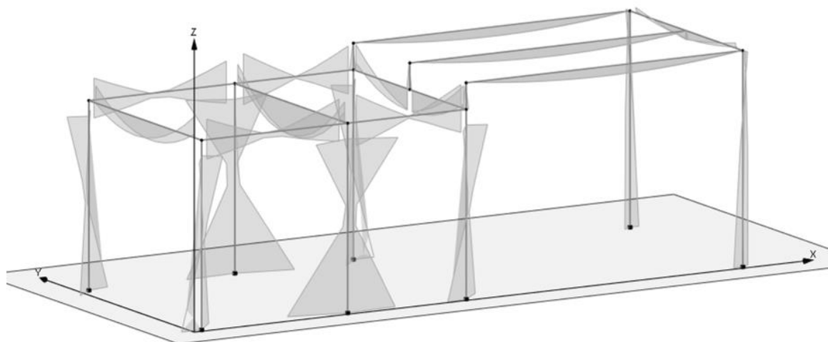
Figura 7.1-4 Diagramma dei momenti M3 – COMB_INV_SLV_CC1
