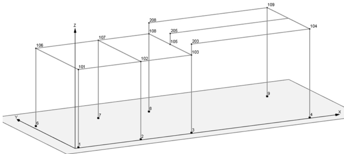
Figura 7.1-2 Numerazione nodi.
