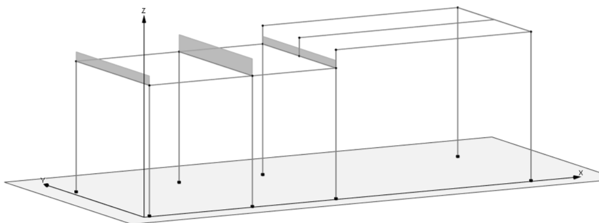
Figura 7.1-11 Schemi di carico – Pesì propri solai
