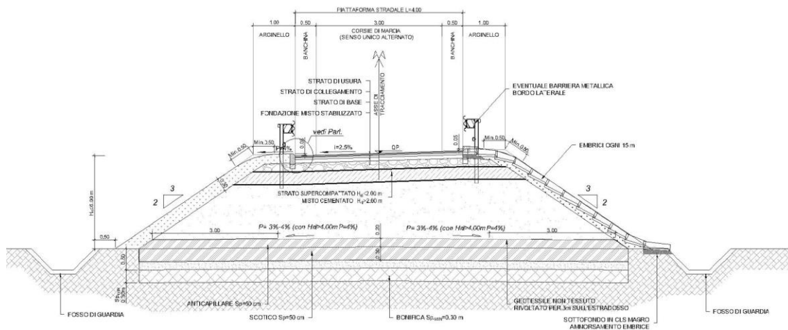
Figure 6-2: sezione tipo strada 4m in rilevato H_{rl} \leq 6.00 m
