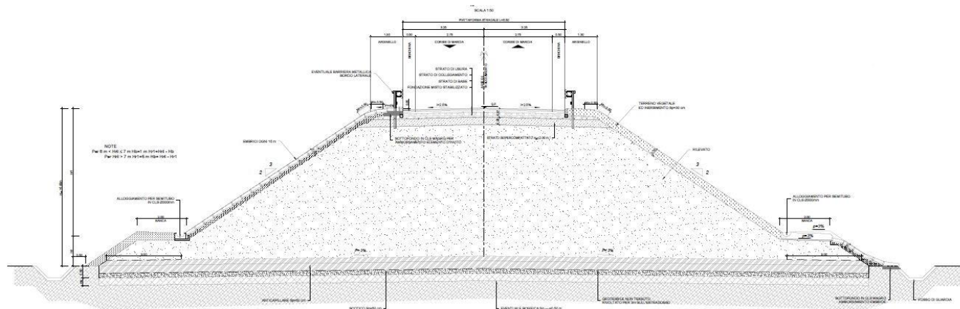
Figure 6-1: Dest. Particolare 6.5m - sezione tipo in rilevato H_{ril} > 6.00 m
