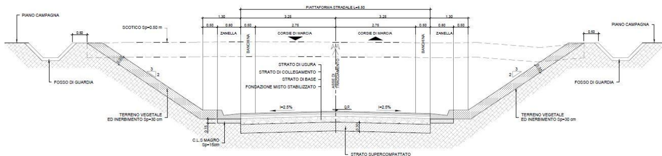
Figure 6-2: Dest. Particolare 6.5m - sezione tipo in trincea
