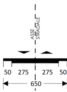
Figura 6-1, NV04B sezione tipo di progetto
