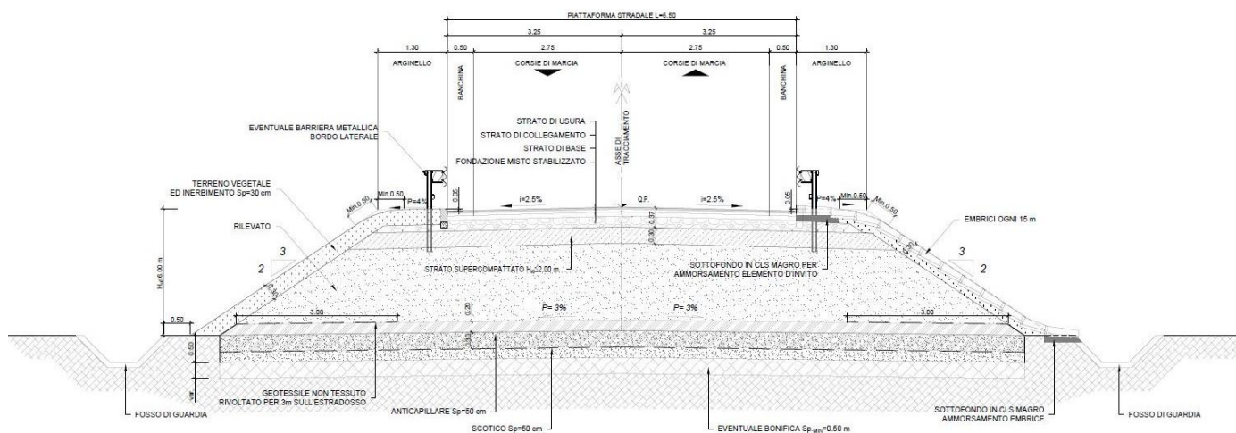
Figura 6-2: Dest. Particolare 6.5m – sezione tipo in rilevato H_{ril} \leq 6.00 m
