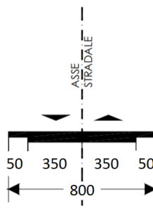
Figura 6-1, NV11B sezione tipo di progetto
