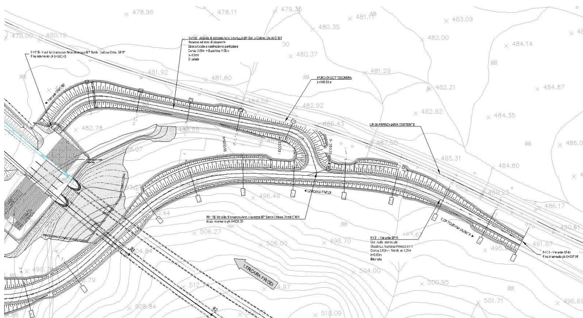
Figure 3-1: stralcio planimetrico NV11 B
