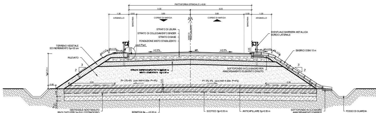
Figure 6-2: sezione tipo strada 8.00m in rilevato H_{ril} \leq 6.00 m
