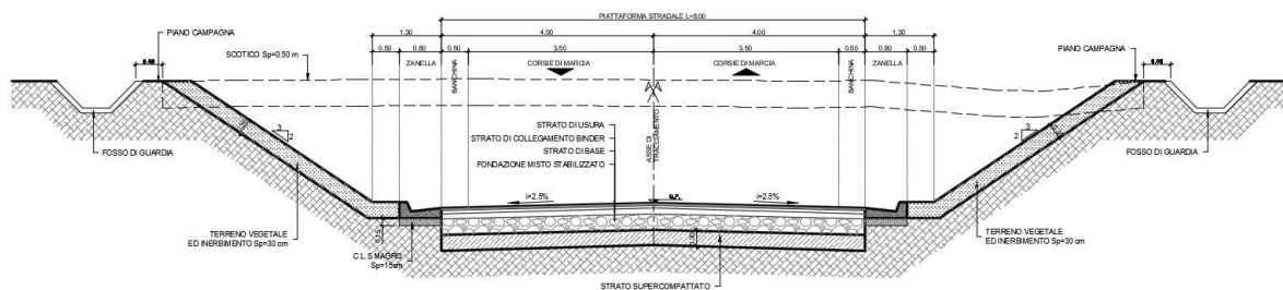
Figure 6-4: sezione tipo strada 4m in trincea
