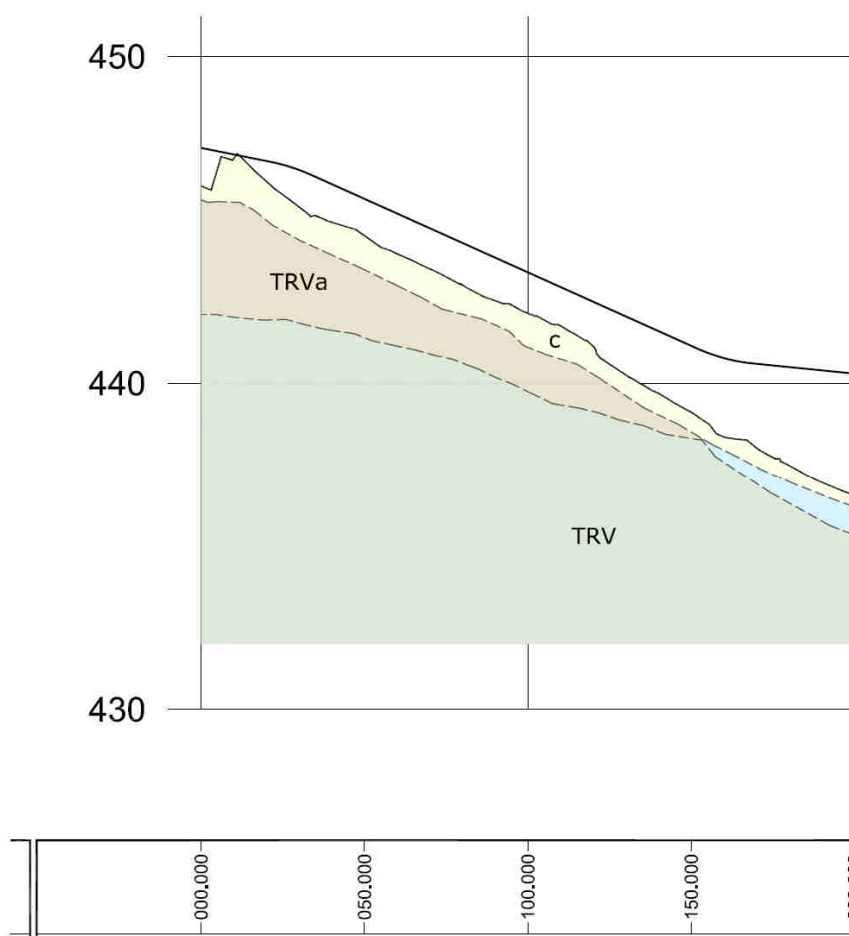
Figura 6-1 – Stralcio del profilo geotecnico.
