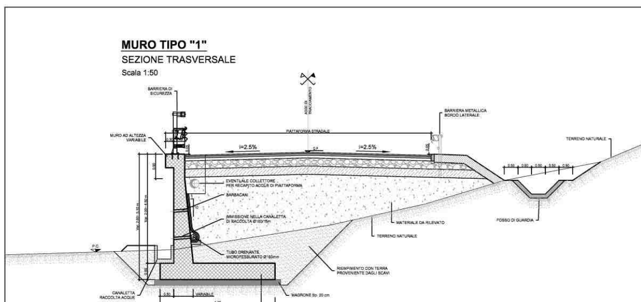
Figura 1-3 – NV07: Muro di sostegno MU19C - Sezione.
