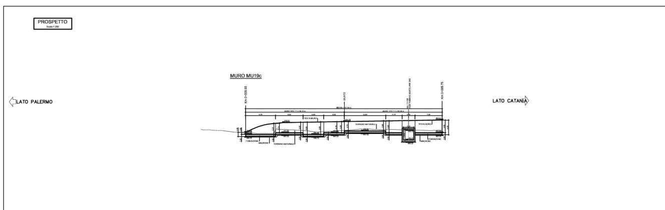
Figura 1-2 – NV07: Muro di sostegno MU19C - Prospetto.
