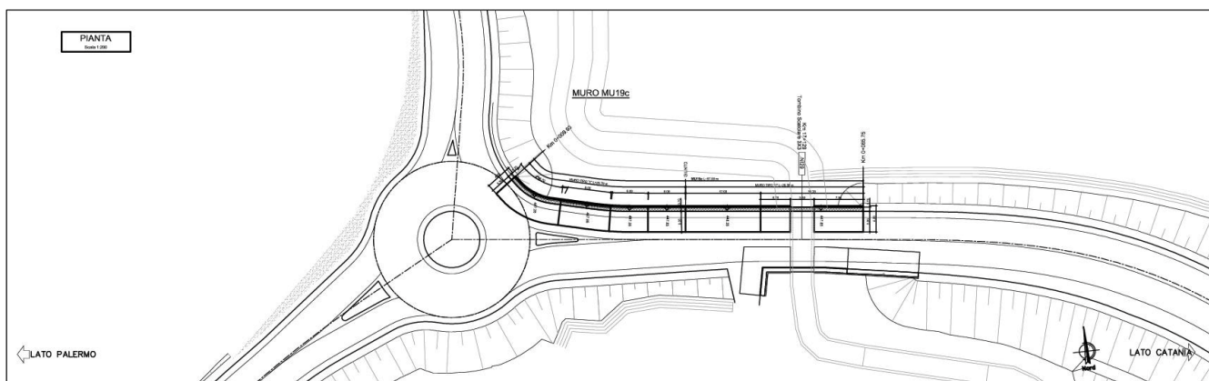
Figura 1-1 – NV07: Muro di sostegno MU19C - Pianta.
