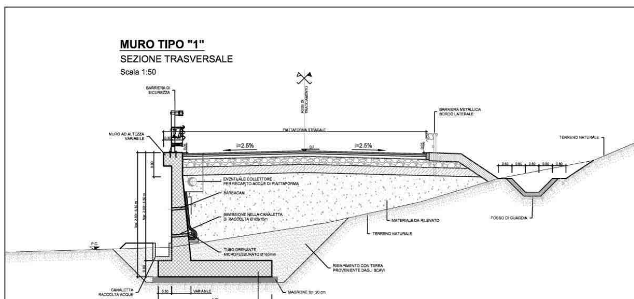
Figura 1-3 – NV07: Muro di sostegno MU19D - Sezione.
