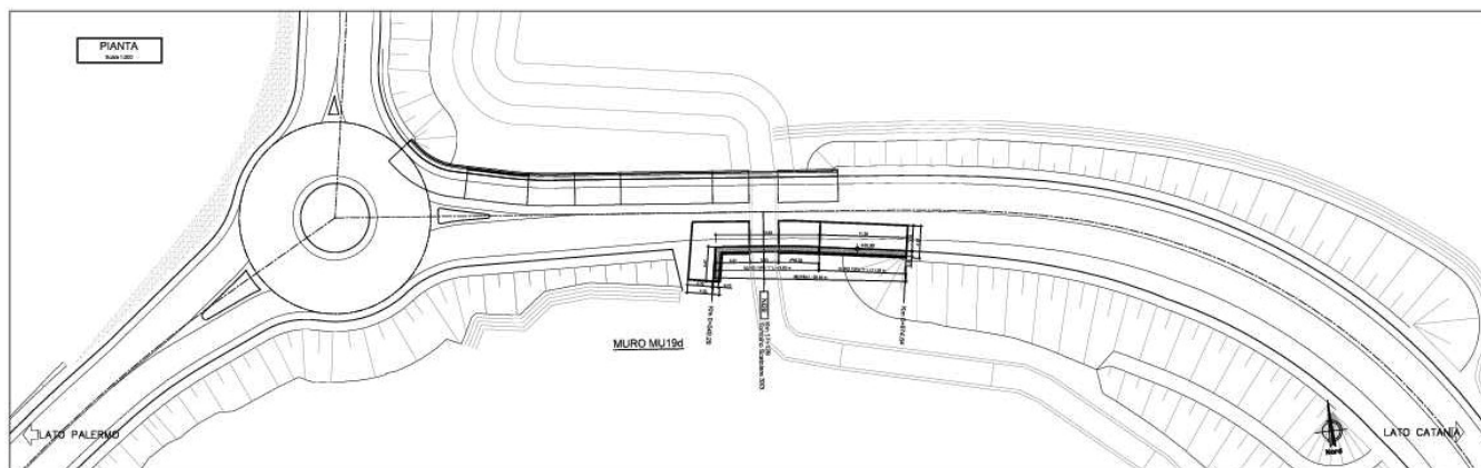
Figura 1-1 – NV07: Muro di sostegno MU19D - Pianta.
