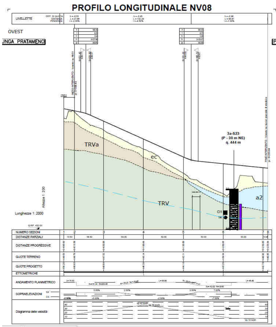
Figura 6-1 – Stralcio del profilo geotecnico.
