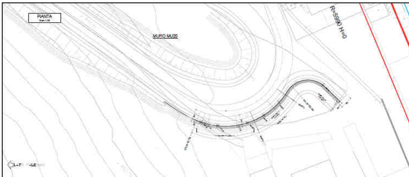
Figura 1-1 – NV08: Muro di sostegno MU20 - Pianta.
