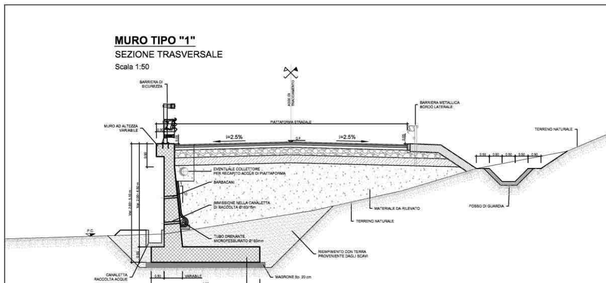
Figura 1-3 – NV08: Muro di sostegno MU20 - Sezione.
