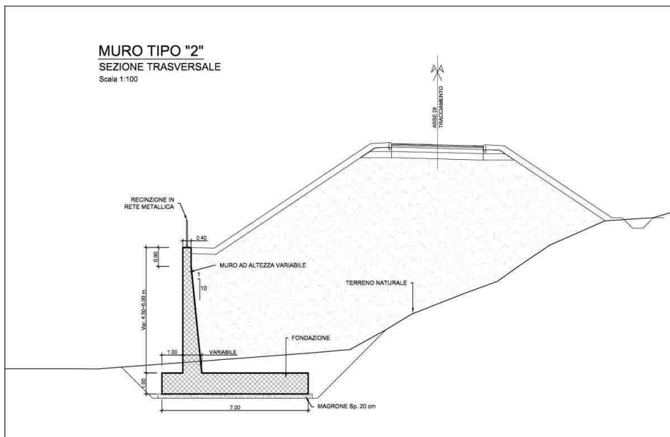
Figura 1-4 – NV11B: Muro di sottoscarpa MU21 – Sezione “tipo 2”
