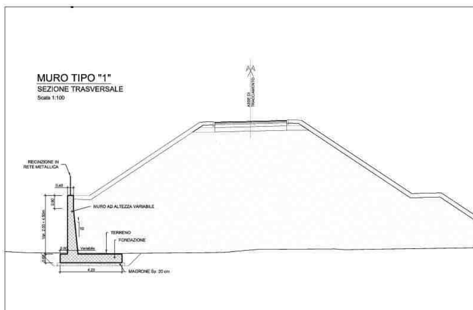
Figura 1-3 – NV11B: Muro di sottoscarpa MU21 – Sezione "tipo 1".
