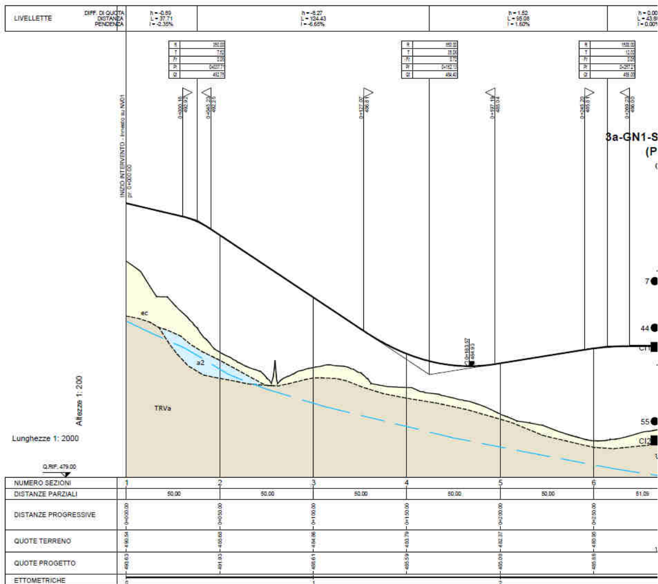
Figura 6-1 – Stralcio del profilo geotecnico.
