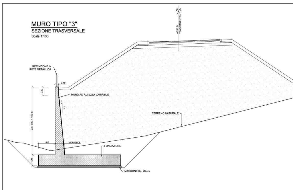
Figura 1-5 – NV11B: Muro di sottoscarpa MU21 – Sezione “tipo 3”
