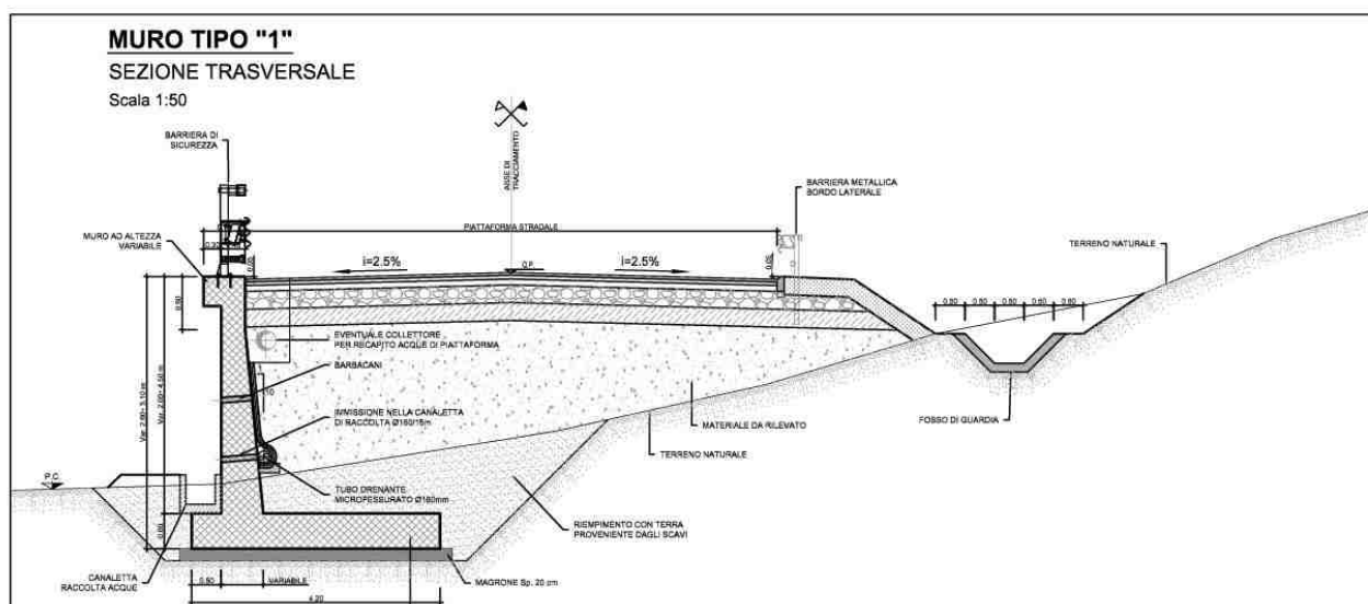
Figura 1-3 – NV01: Muro di sostegno MU17H – Sezione trasversale muro tipo 1.
