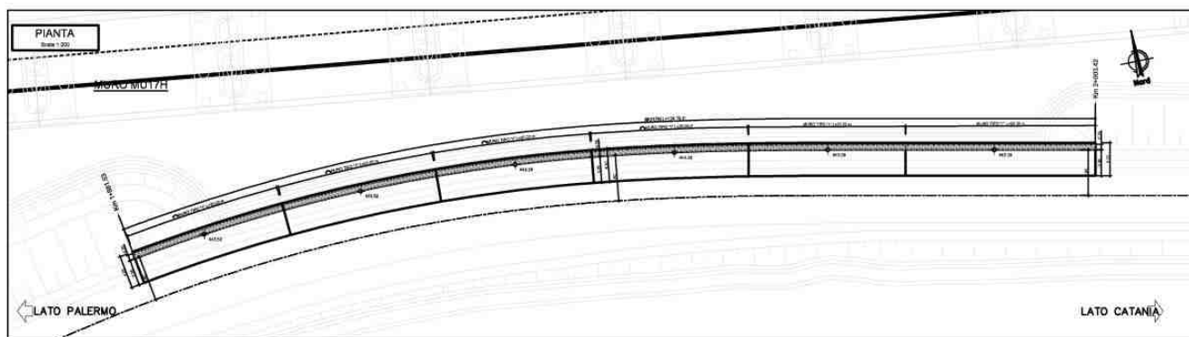
Figura 1-1 – NV01: Muro di sostegno MU17H - Pianta.
