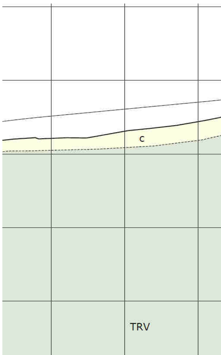
Figura 6-1 – Stralcio del profilo geotecnico.
