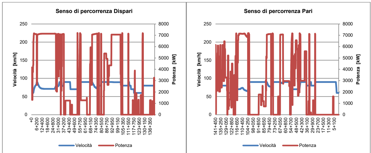
Figura 6 – Mercì "E186" – Diagrammi Spazio/Velocità - Spazio/Potenza
