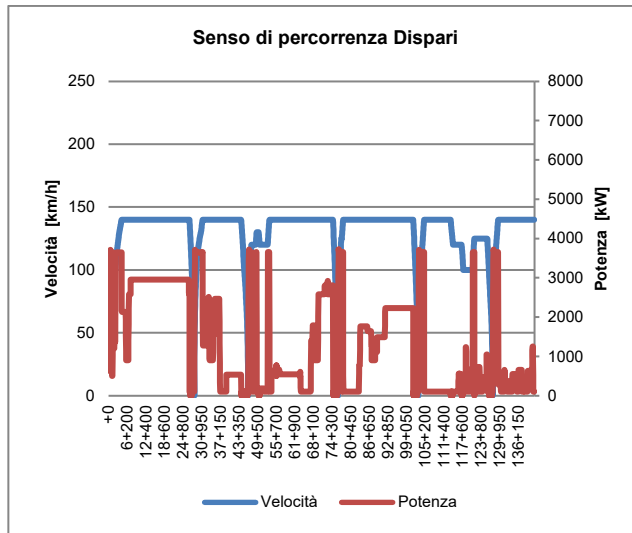
Figura 3 – Regionale "E464" – Diagrammi Spazio/Velocità - Spazio/Potenza
