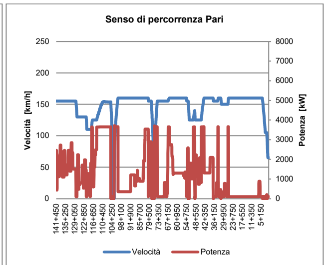
Figura 4 – Regionale Veloce "E464" – Diagrammi Spazio/Velocità - Spazio/Potenza
