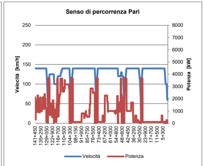
Figura 3 – Regionale "E464" – Diagrammi Spazio/Velocità - Spazio/Potenza
