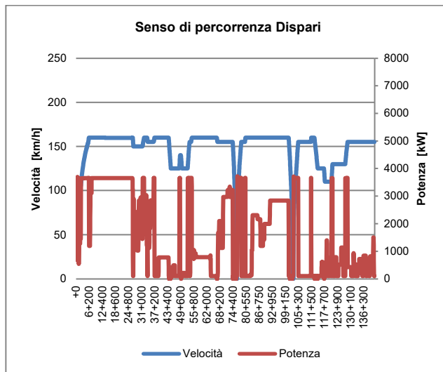
Figura 4 – Regionale Veloce "E464" – Diagrammi Spazio/Velocità - Spazio/Potenza
