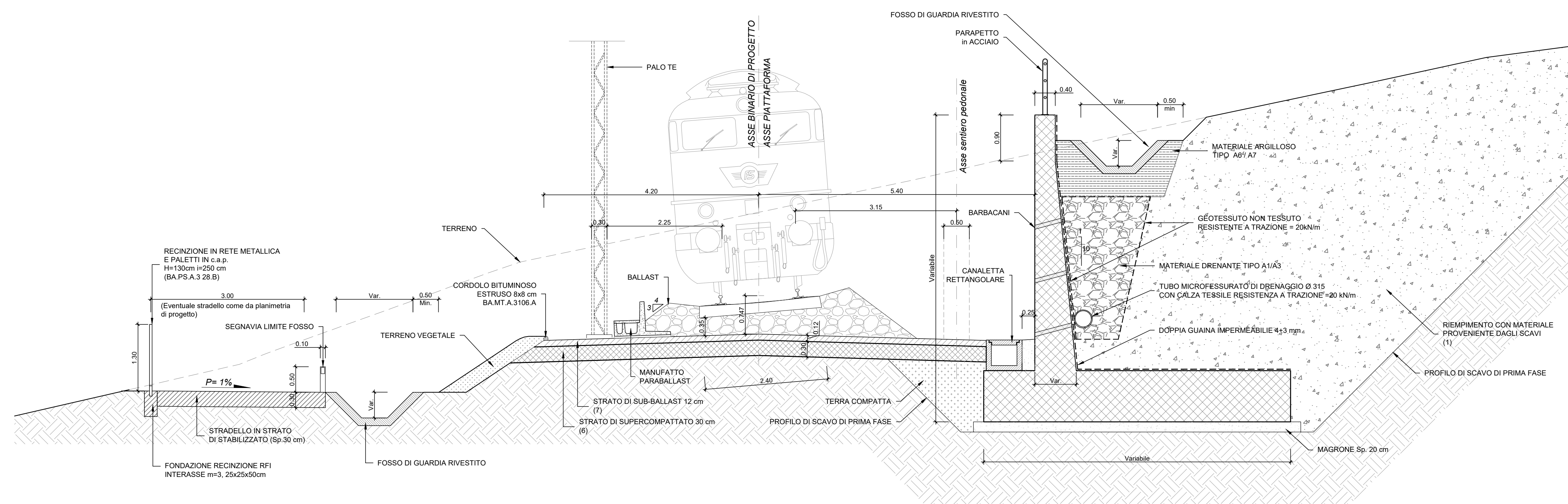
SEZIONE TIPO TRINCEA a singolo binario in curva con muro a mensola di controripa SCALA 1:50
