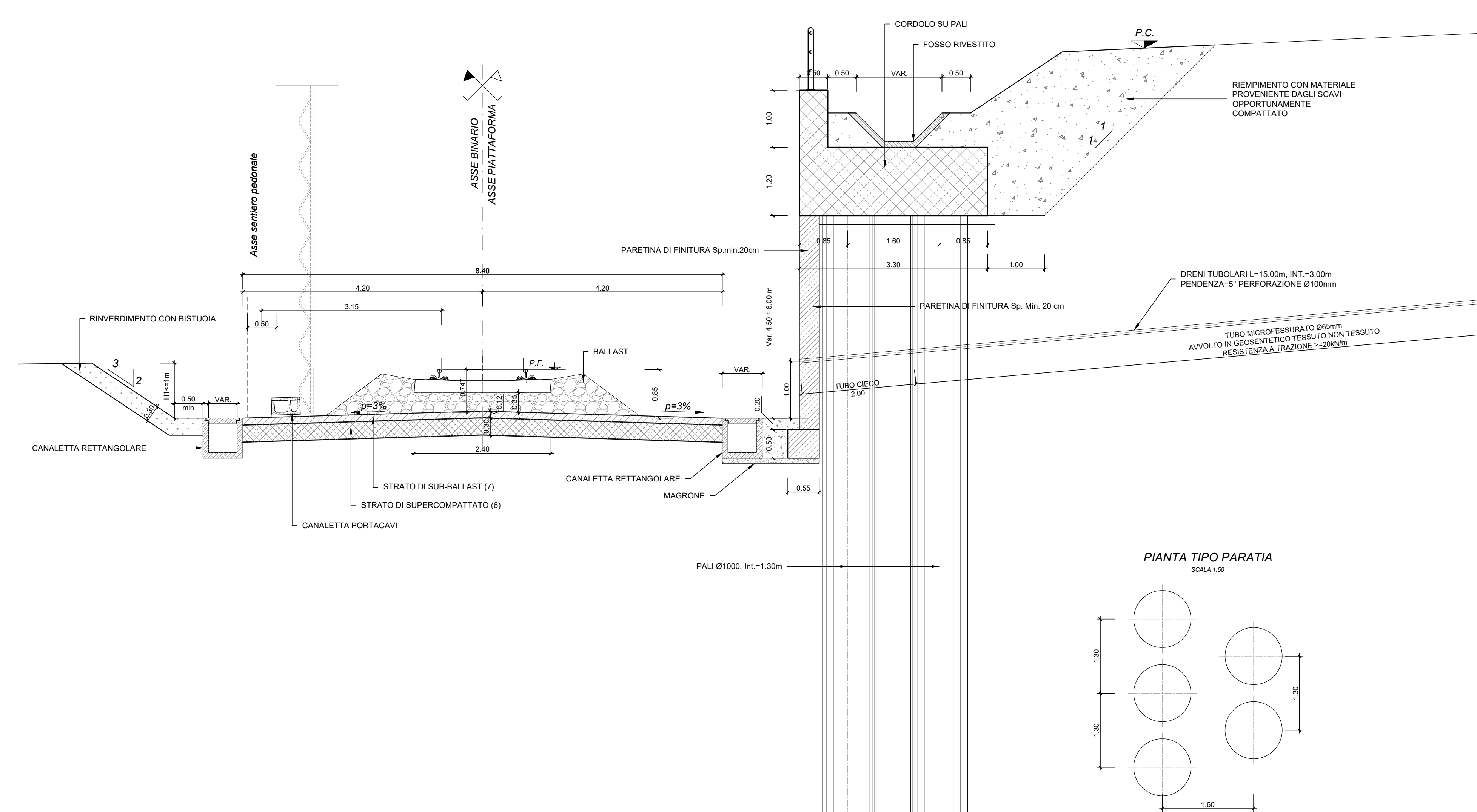
TRINCEE PER H > 4.0m CON PARATIA TIPO C IN DX SCALA 1:50
