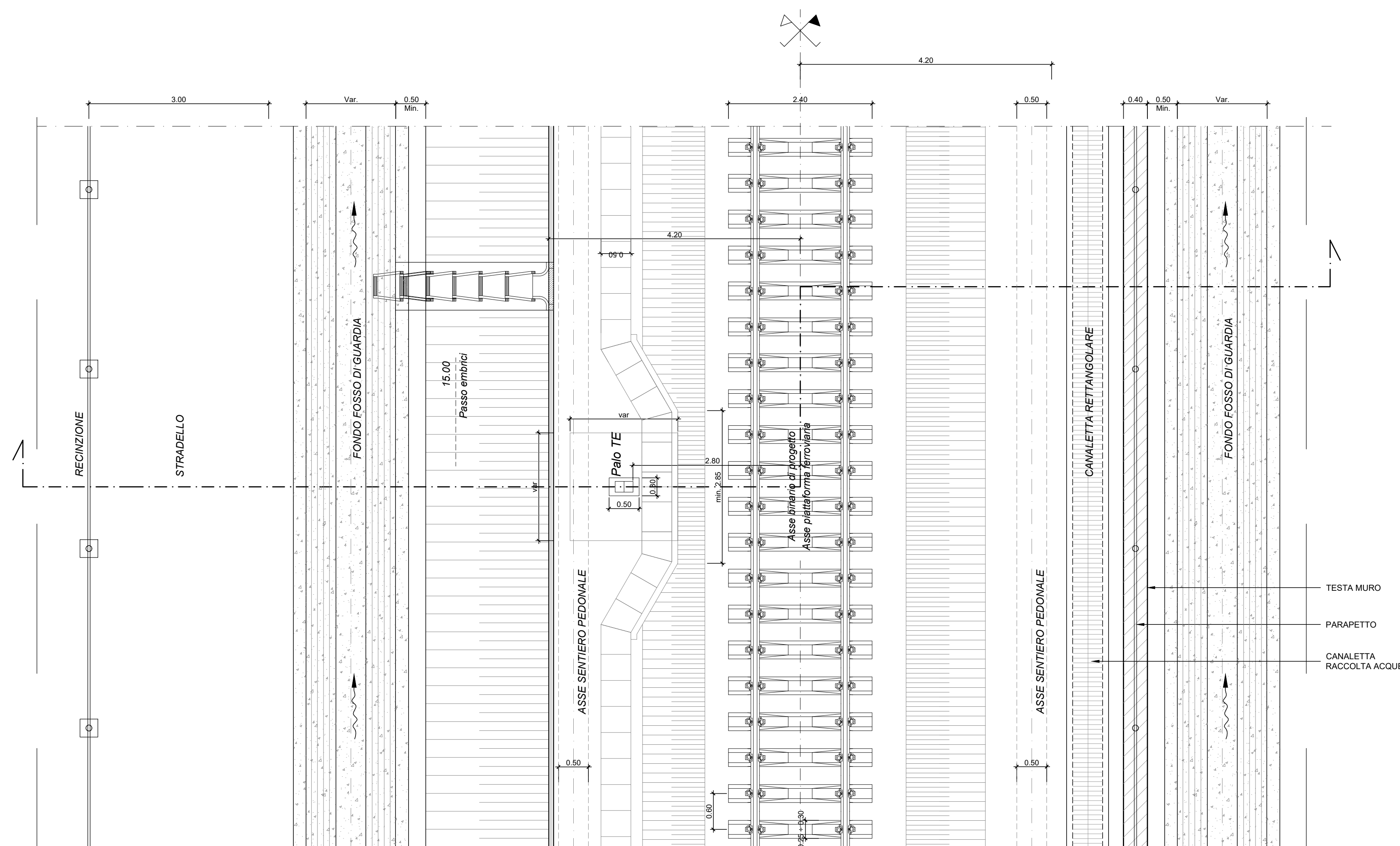
SEZIONE TIPO TRINCEA Pianta per sezione a singolo binario in curva con muro a mensola di controripa SCALA 1:50
