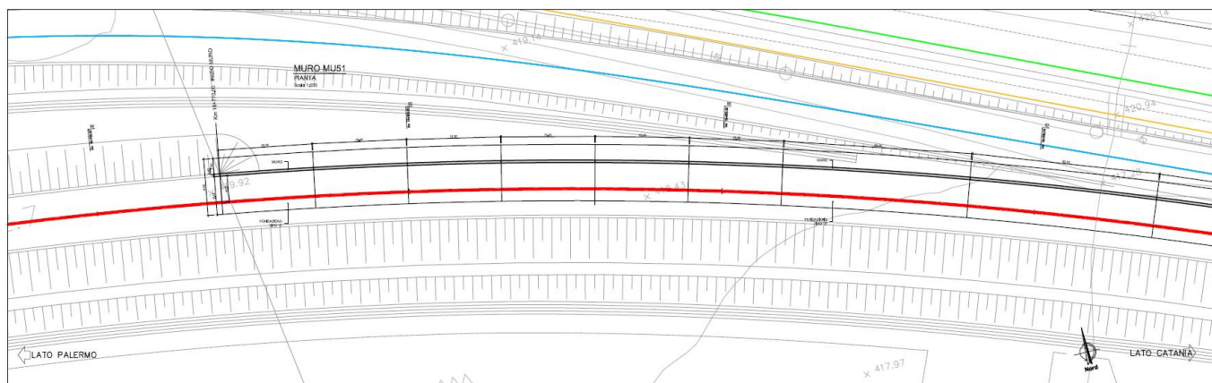
Figura 1-1 – RI08: Muro di sostegno in sx MU51 - Pianta.
