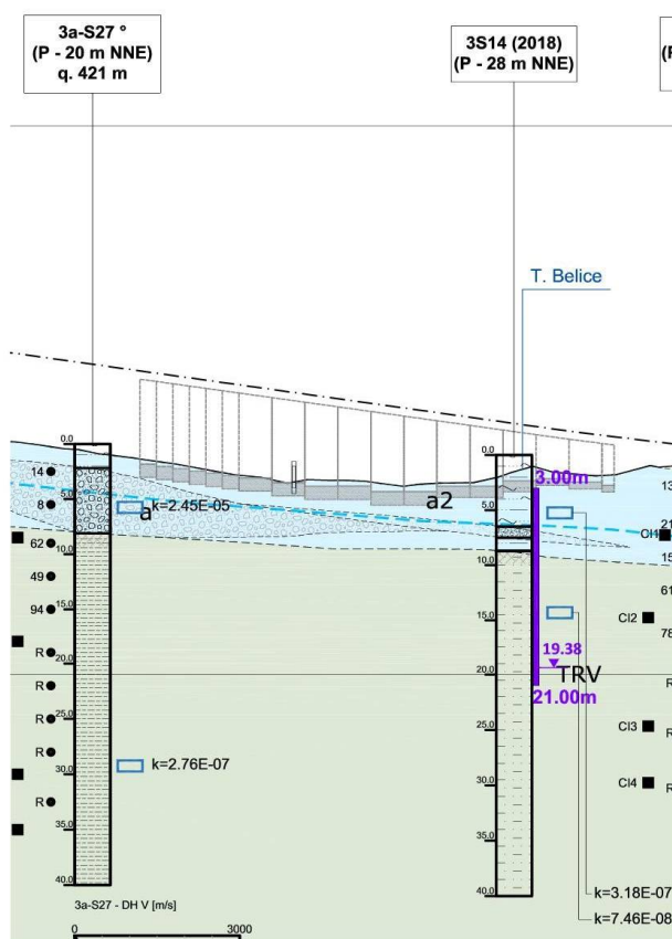
Figura 6-1 – Stralcio del profilo geotecnico.
