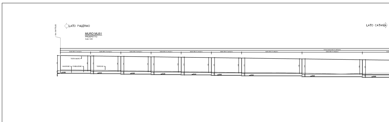
Figura 1-4 – RI08: Muro di sostegno in sx MU51 - Prospetto.
