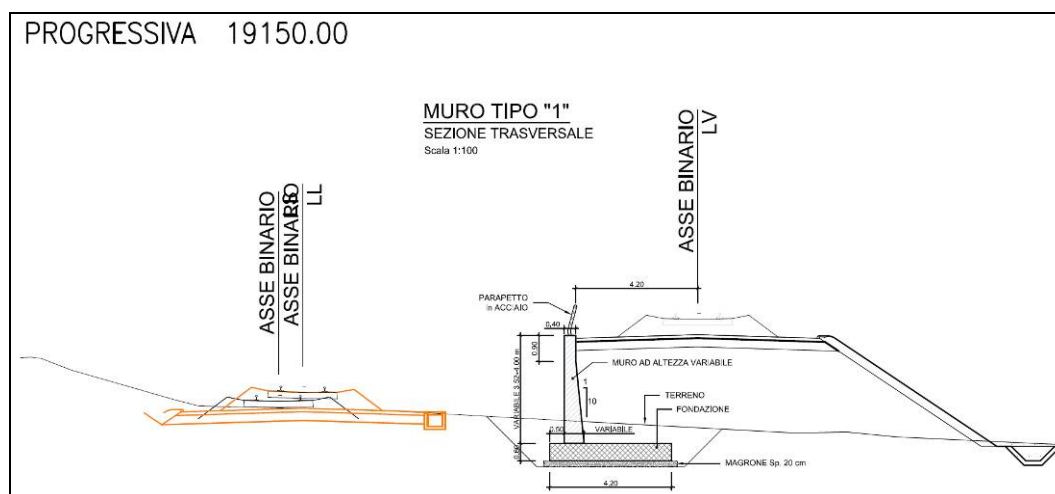
Figura 1-7 – RI08: Muro di sostegno in sx MU51 – Sezione trasversale muro tipo 1.
