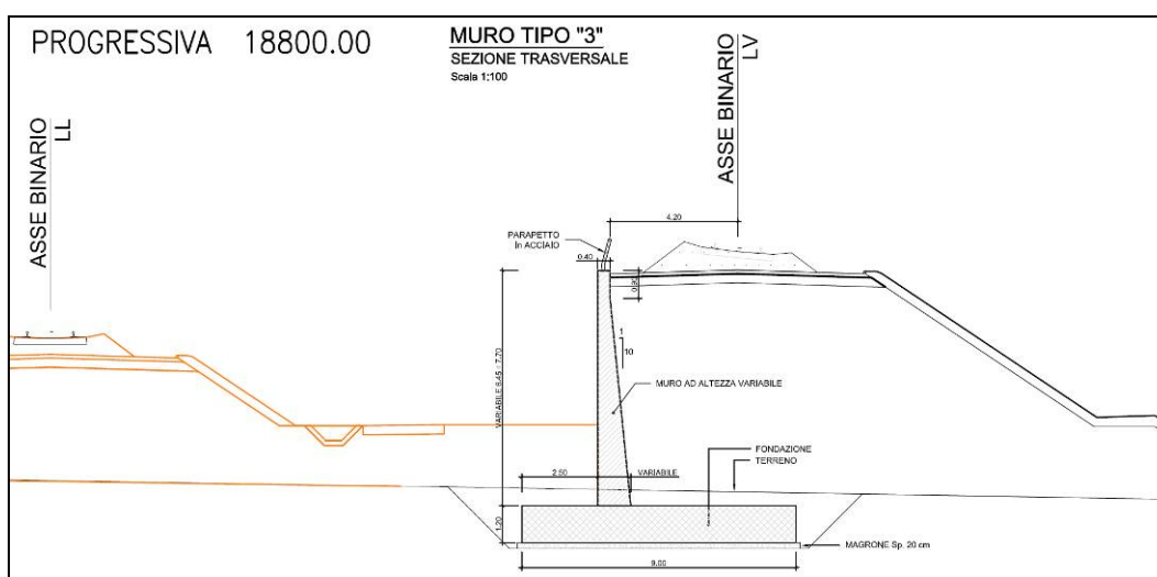
Figura 1-9 – RI08: Muro di sostegno in sx MU51 – Sezione trasversale muro tipo 3.
