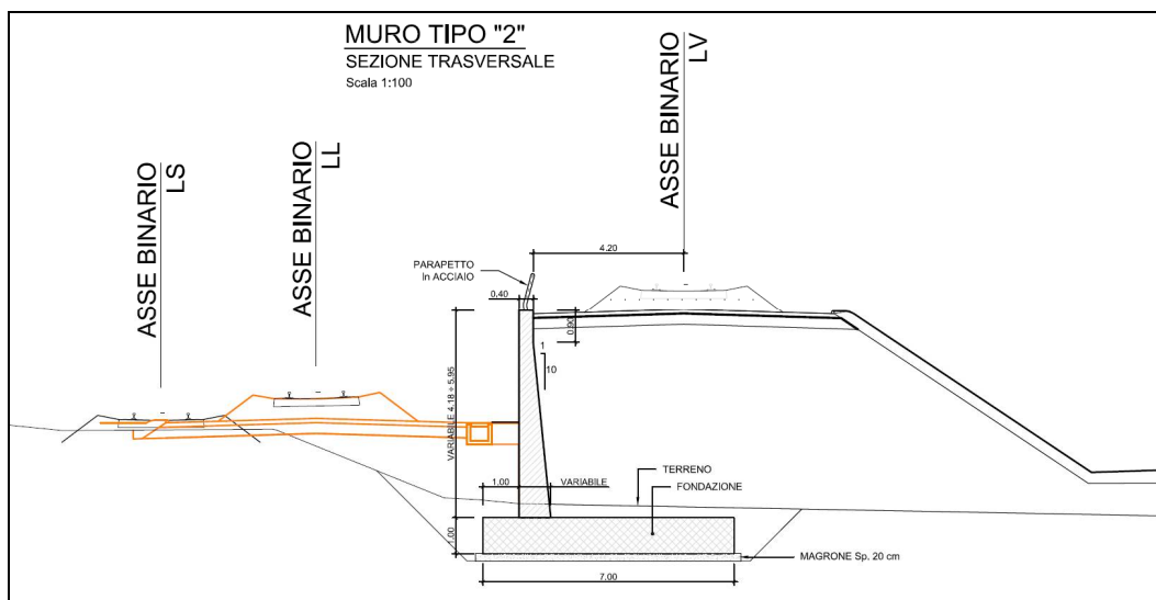
Figura 1-8 – RI08: Muro di sostegno in sx MU51 – Sezione trasversale muro tipo 2.
