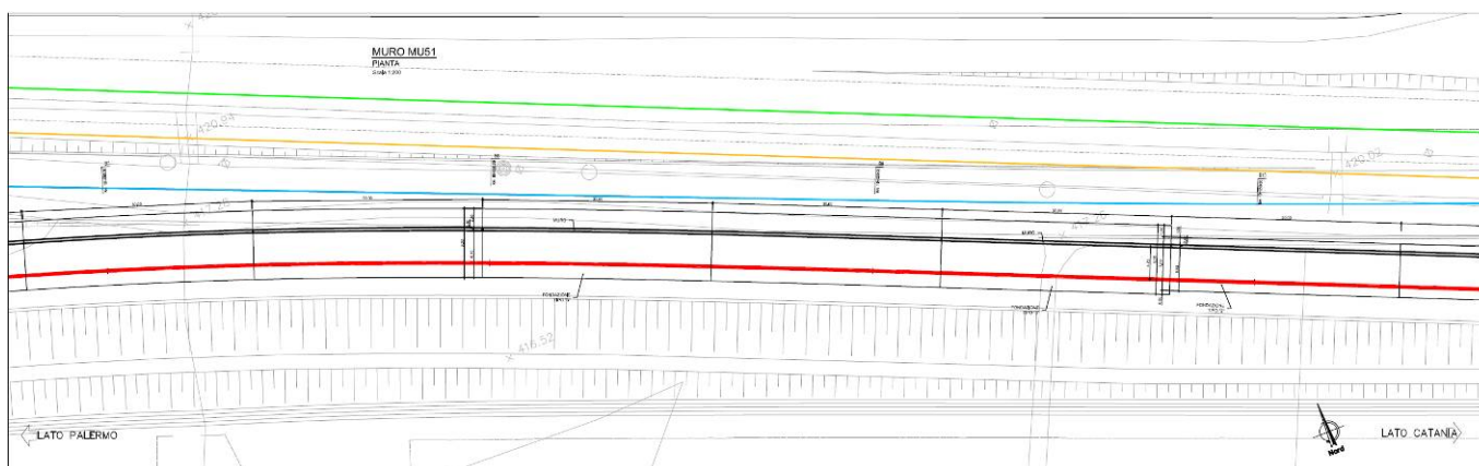
Figura 1-2 – RI08: Muro di sostegno in sx MU51 - Pianta.
