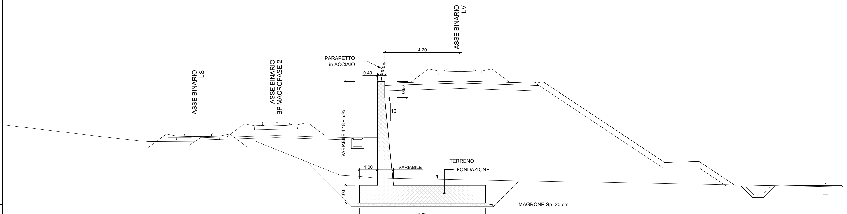
MURO TIPO "2" SEZIONE TRASVERSALE - PK. 19+038.90 + 19+128.90 Scala 1:100
