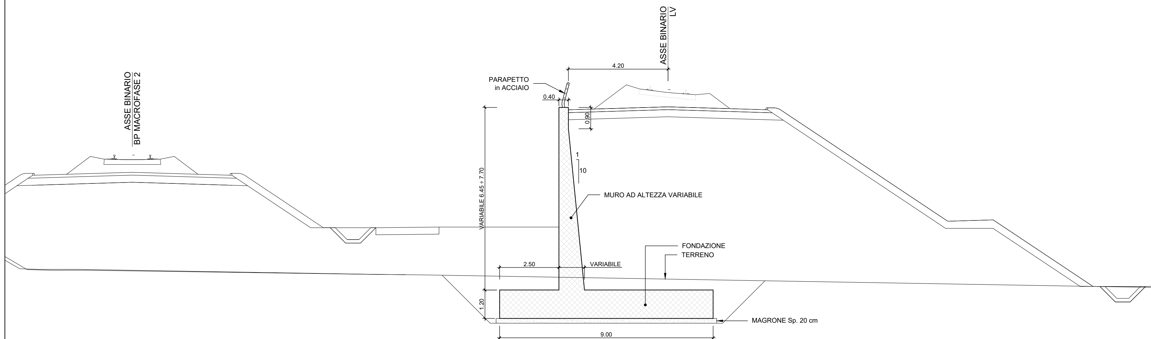
MURO TIPO "3" SEZIONE TRASVERSALE - PK. 18+770.00 + 19+038.90 Scala 1:100
