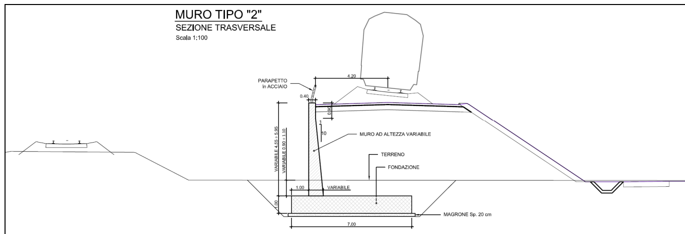
Figura 1-5 – RI08: Muro di sostegno in sx MU52 – Sezione trasversale muro tipo 2.
