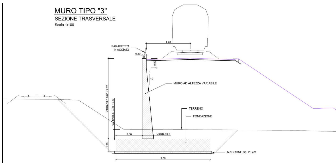
Figura 1-6 – RI08: Muro di sostegno in sx MU52 – Sezione trasversale muro tipo 3.
