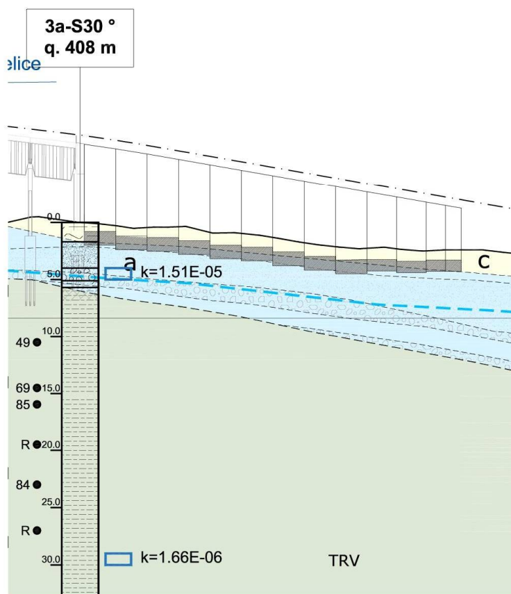
Figura 6-1 – Stralcio del profilo geotecnico.
