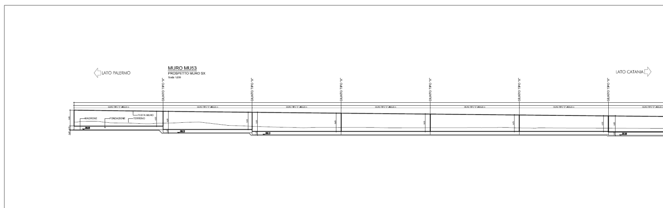
Figura 1-4 – RI09: Muro di sostegno in sx MU53 - Prospetto.
