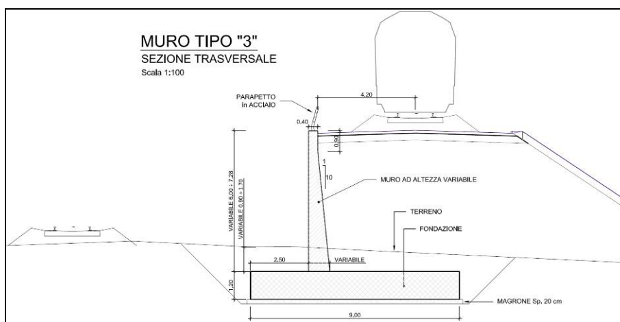
Figura 1-8 – RI08: Muro di sostegno in sx MU53 – Sezione trasversale muro tipo 3.
