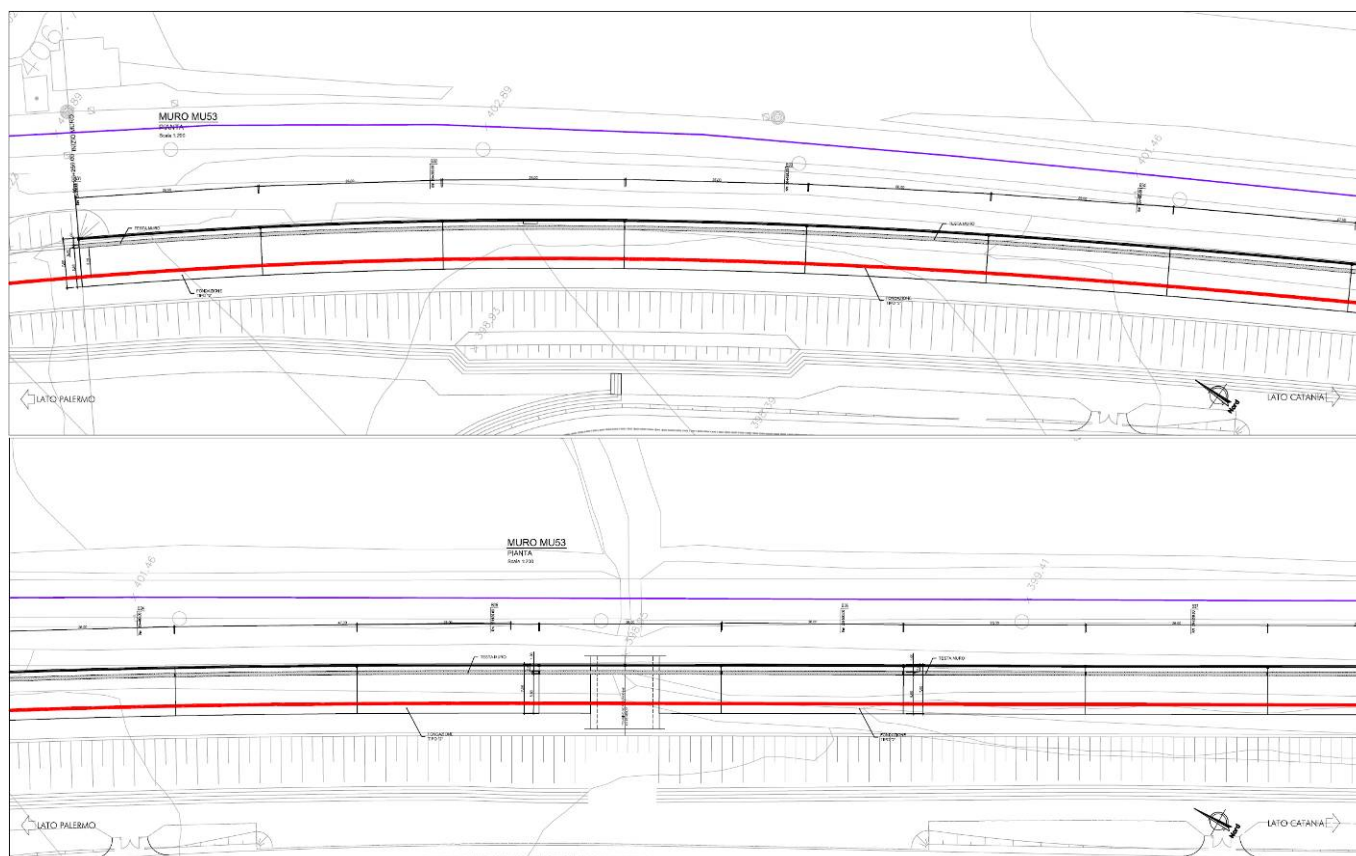
Figura 1-1 – RI09: Muro di sostegno in sx MU53 - Pianta.
