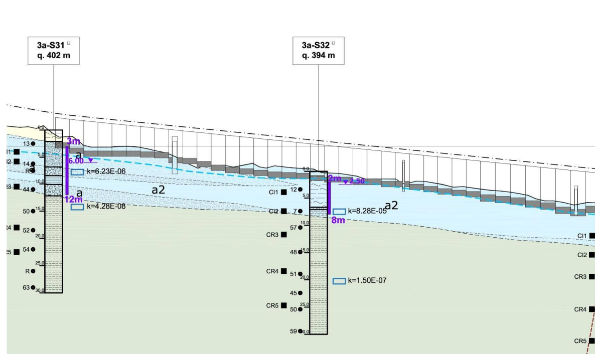
Figura 6-1 – Stralcio del profilo geotecnico.
