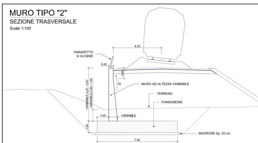
Figura 1-7 – RI08: Muro di sostegno in sx MU53 – Sezione trasversale muro tipo 2.
