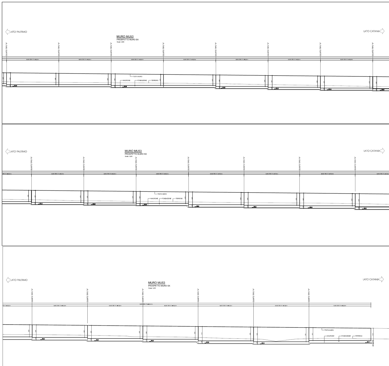
Figura 1-6 – RI09: Muro di sostegno in sx MU53 - Prospetto.
