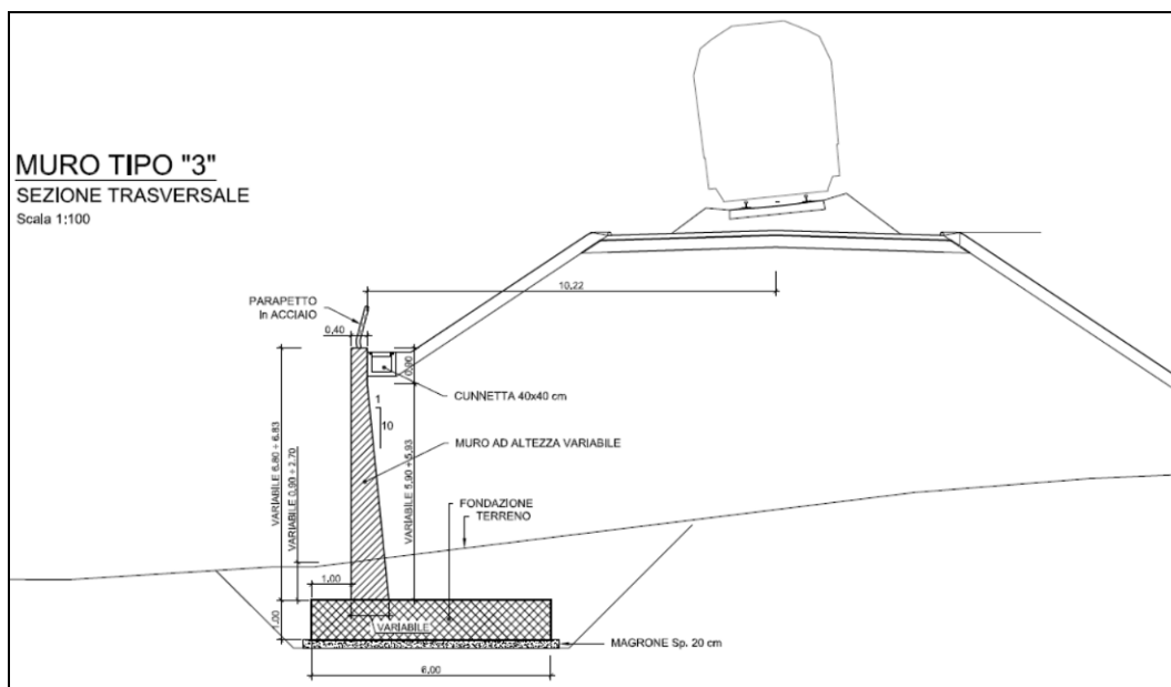
Figura 1-6 – RI10: Muro di sostegno in sx MU54 – Sezione trasversale muro tipo 3.
