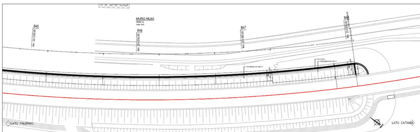
Figura 1-2 – RI10: Muro di sostegno in sx MU54 - Pianta.
