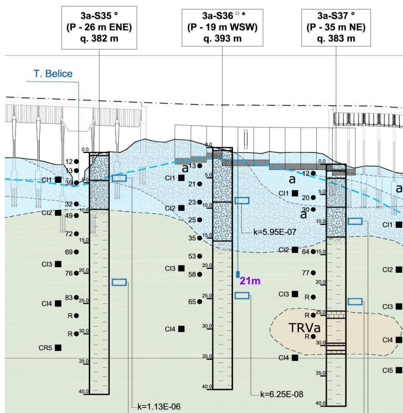
Figura 6-1 – Stralcio del profilo geotecnico.
