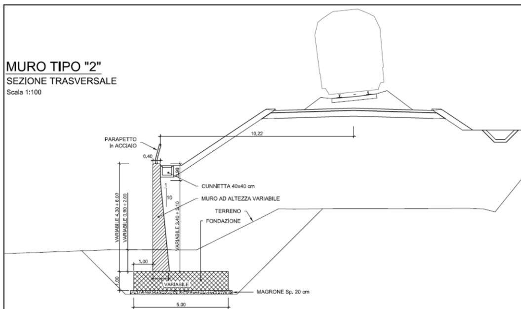
Figura 1-5 – RI10: Muro di sostegno in sx MU54 – Sezione trasversale muro tipo 2.
