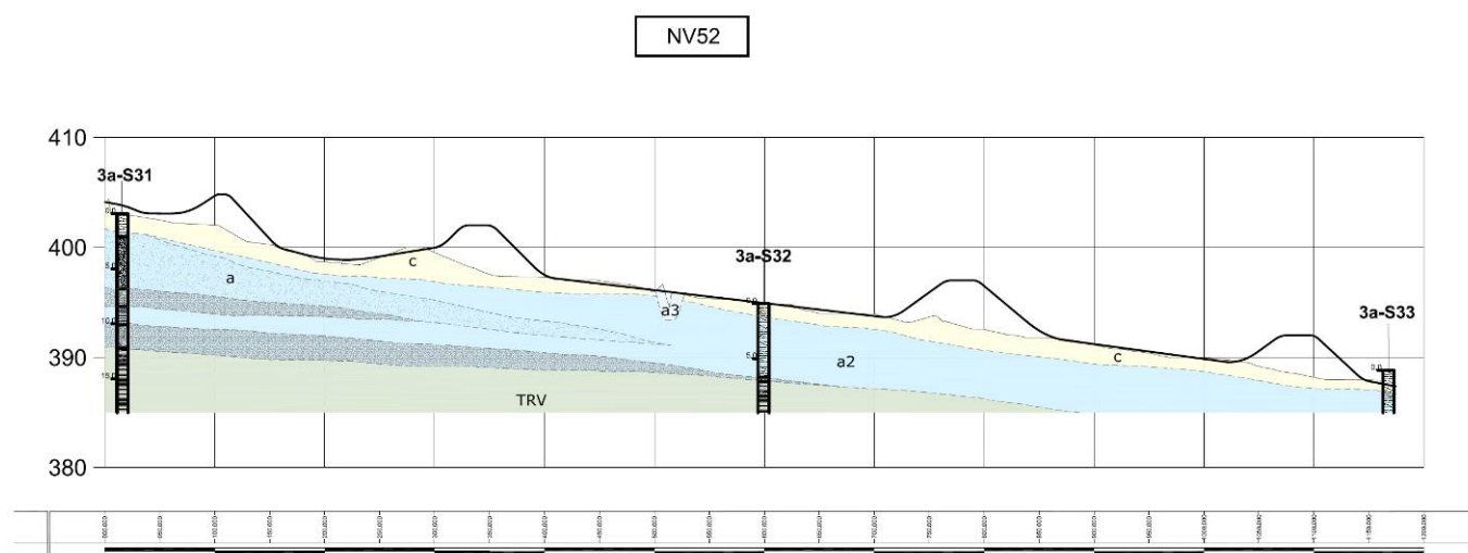
Figura 6-1 – Stralcio del profilo geotecnico.
