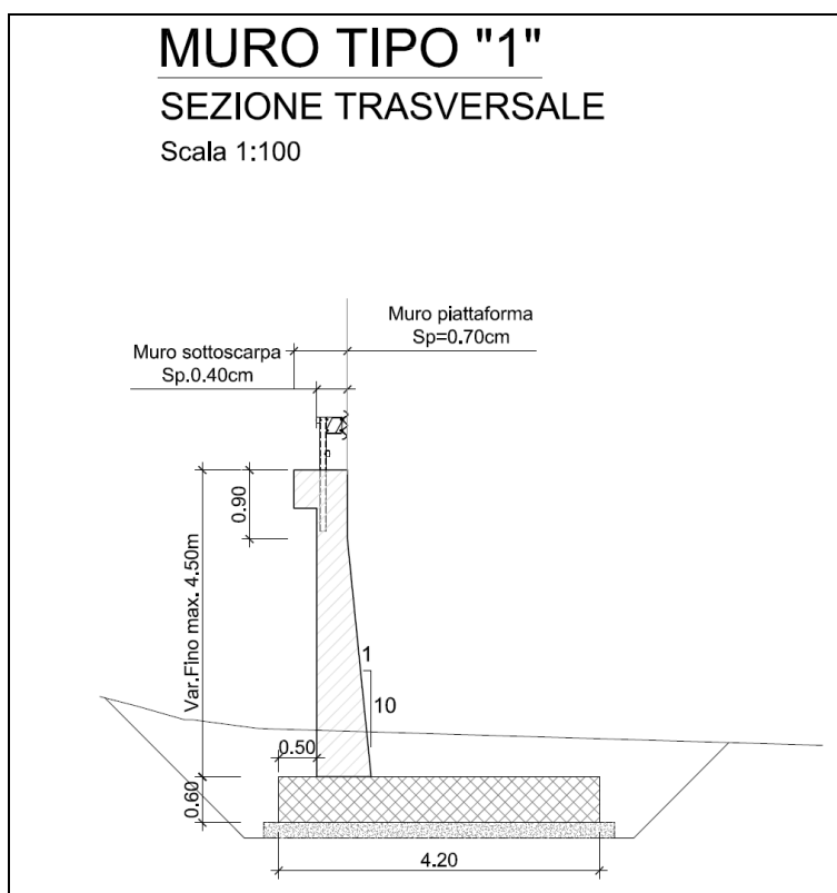
Figura 1-3 – NV52: Muro di sostegno MU79A - Sezione.
