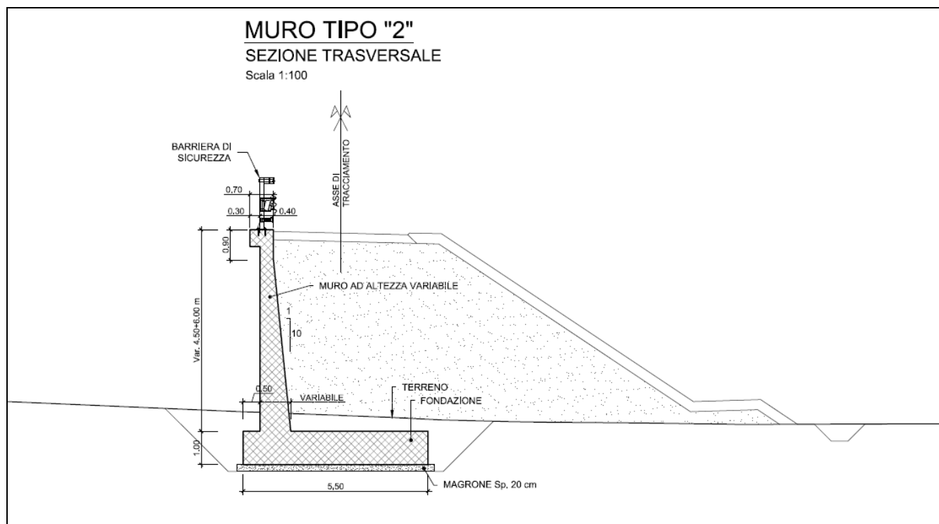
Figura 1-4 – NV52: Muro di sostegno MU79A - Sezione.
