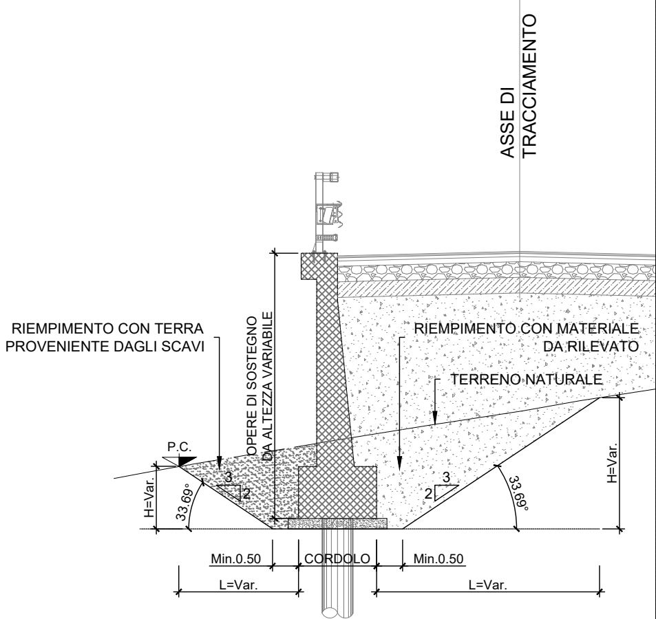
SEZION TIPO SEZIONE TRASVERSALE Scala 1:100
