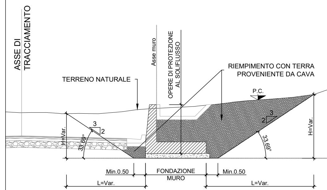
SEZIONE TIPO SEZIONE TRASVERSALE Scala 1:100
