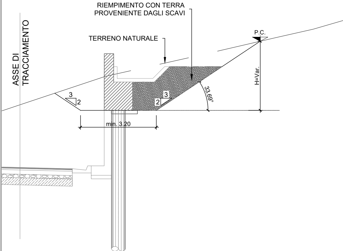
SEZIONE TIPO SEZIONE TRASVERSALE Scala 1:100
