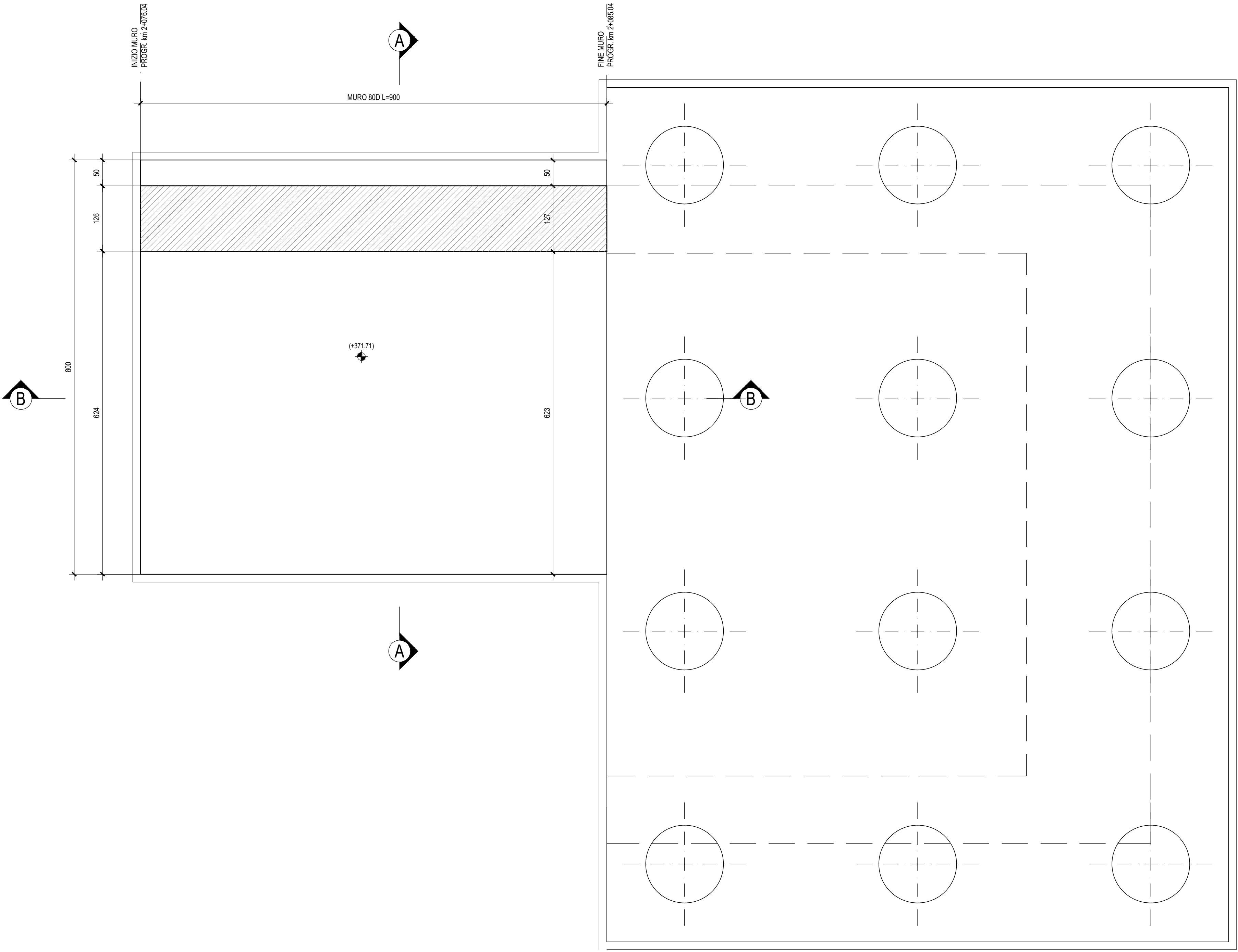
PIANTA SPICCATO - Scala 1:50
