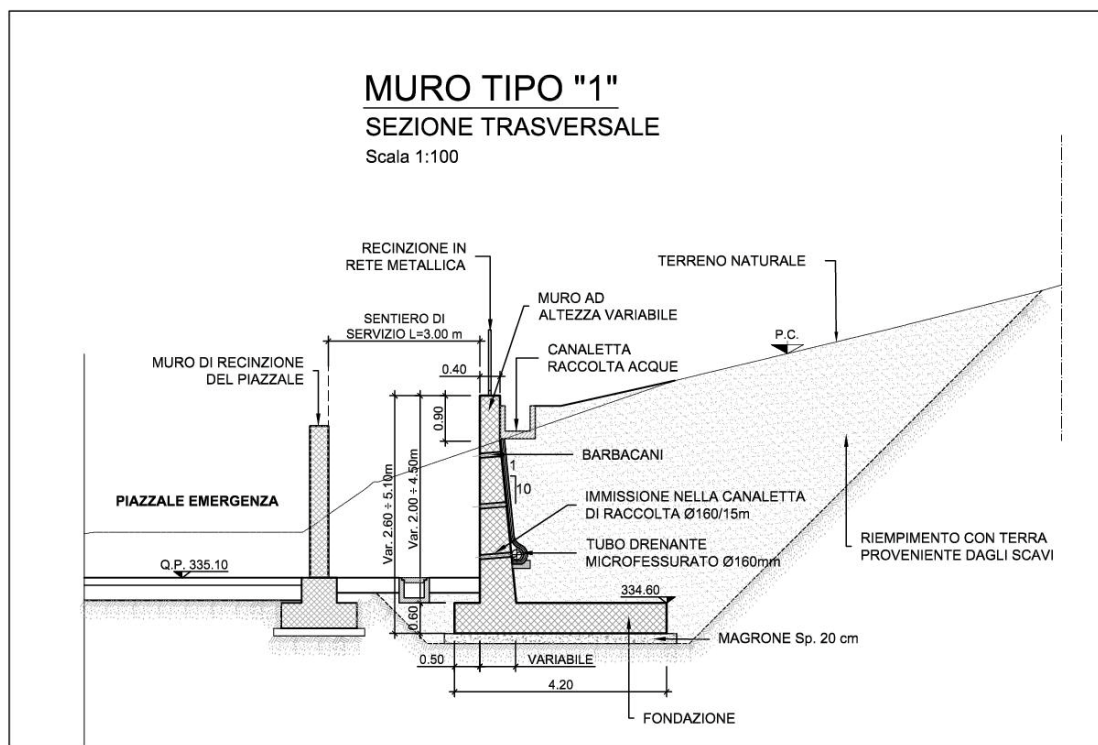
Figura 1-3 – PT57: Muro di sostegno MU90B - Sezione.
