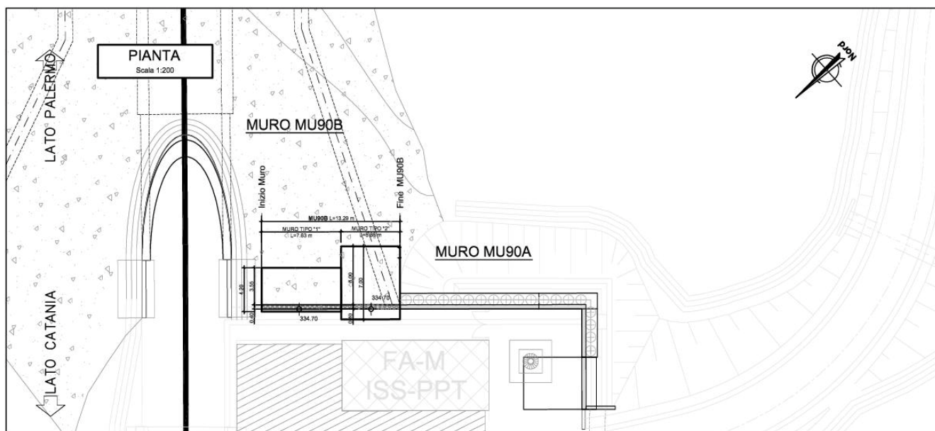
Figura 1-1 – PT57: Muro di sostegno MU90B - Pianta.
