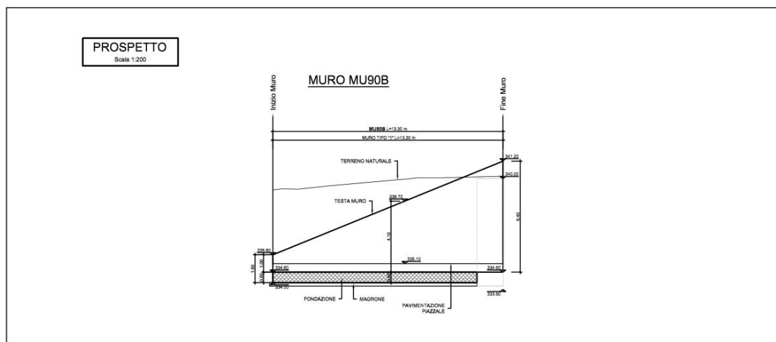
Figura 1-2 – PT57: Muro di sostegno MU90B - Prospetto.
