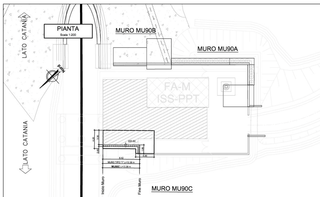
Figura 1-1 – PT57: Muro di sostegno MU90C - Pianta.
