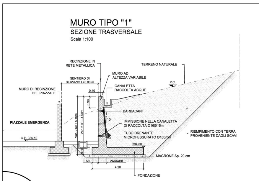
Figura 1-3 – PT57: Muro di sostegno MU90B - Sezione.
