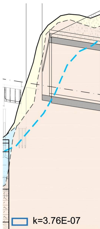
Figura 6-1 – Stralcio del profilo geotecnico.
