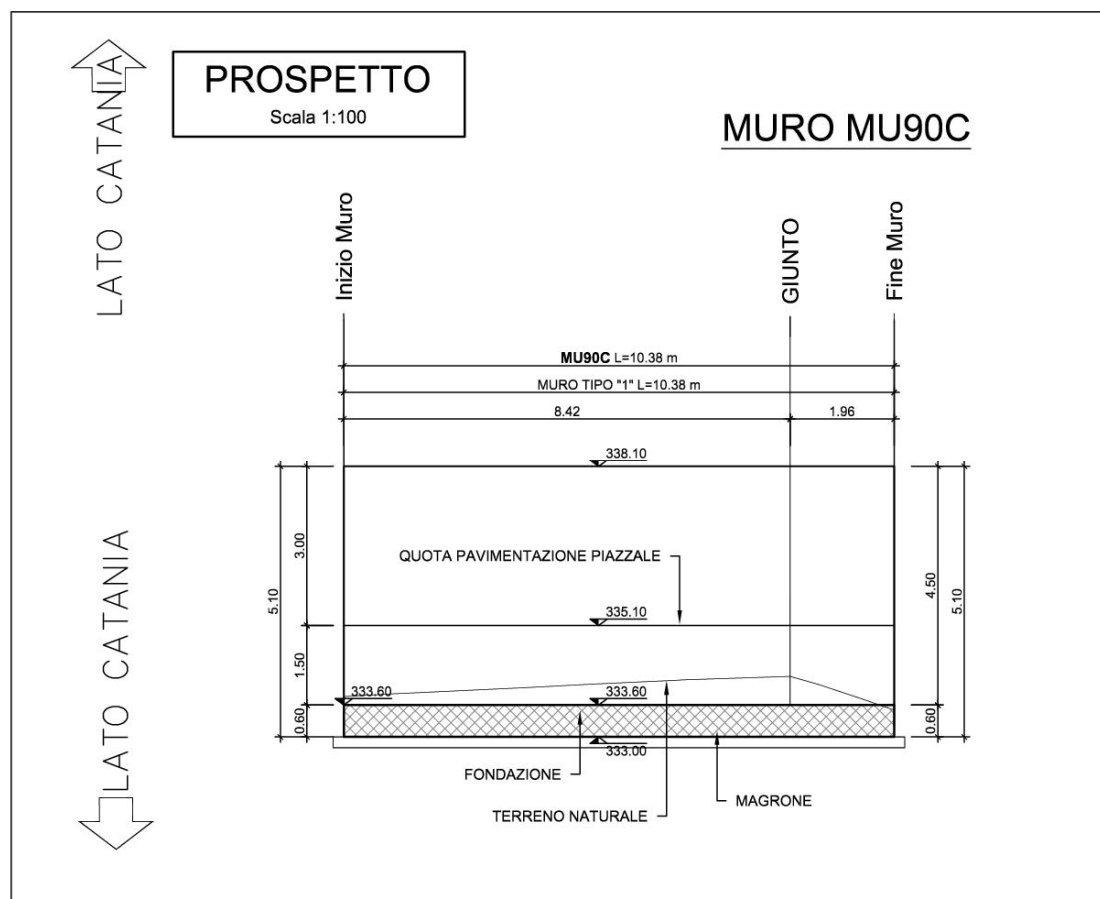
Figura 1-2 – PT57: Muro di sostegno MU90C - Prospetto.
