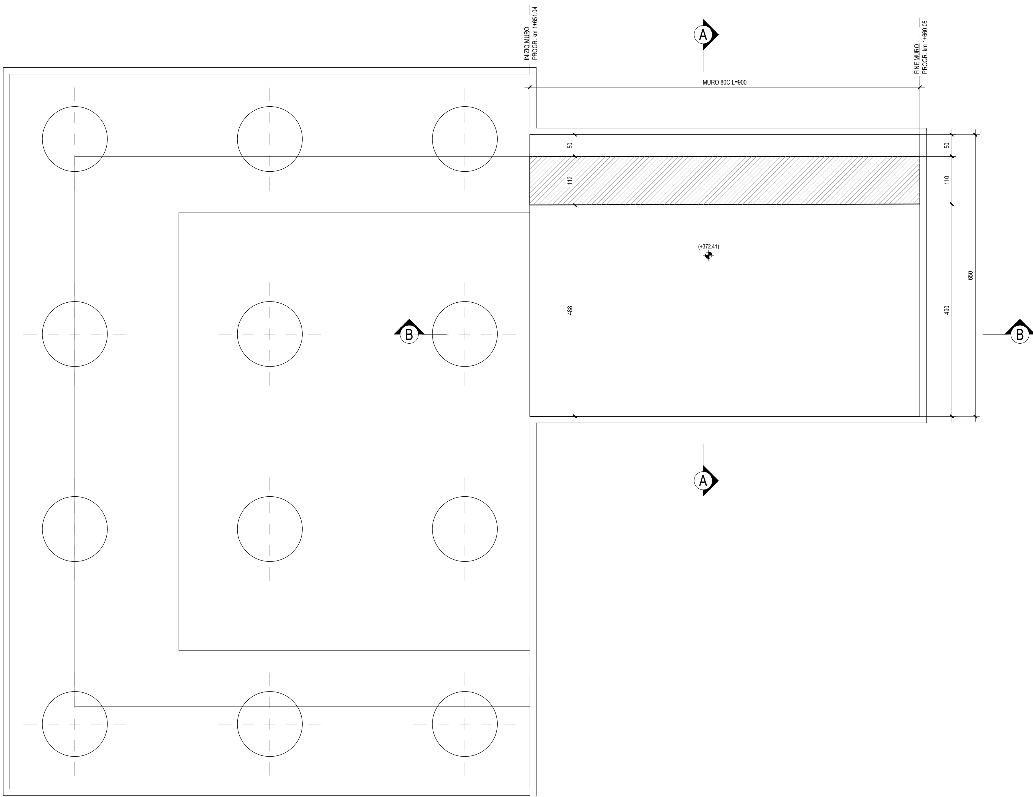
PIANTA SPICCATO - Scala 1:50
