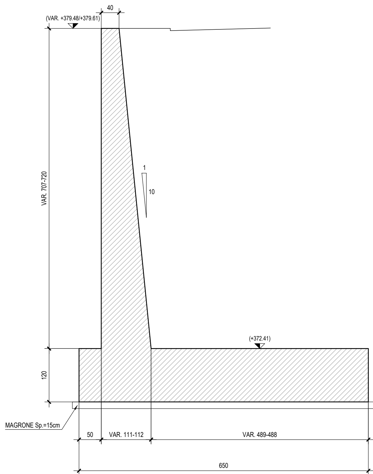
SEZIONE A-A - Scala 1:50
