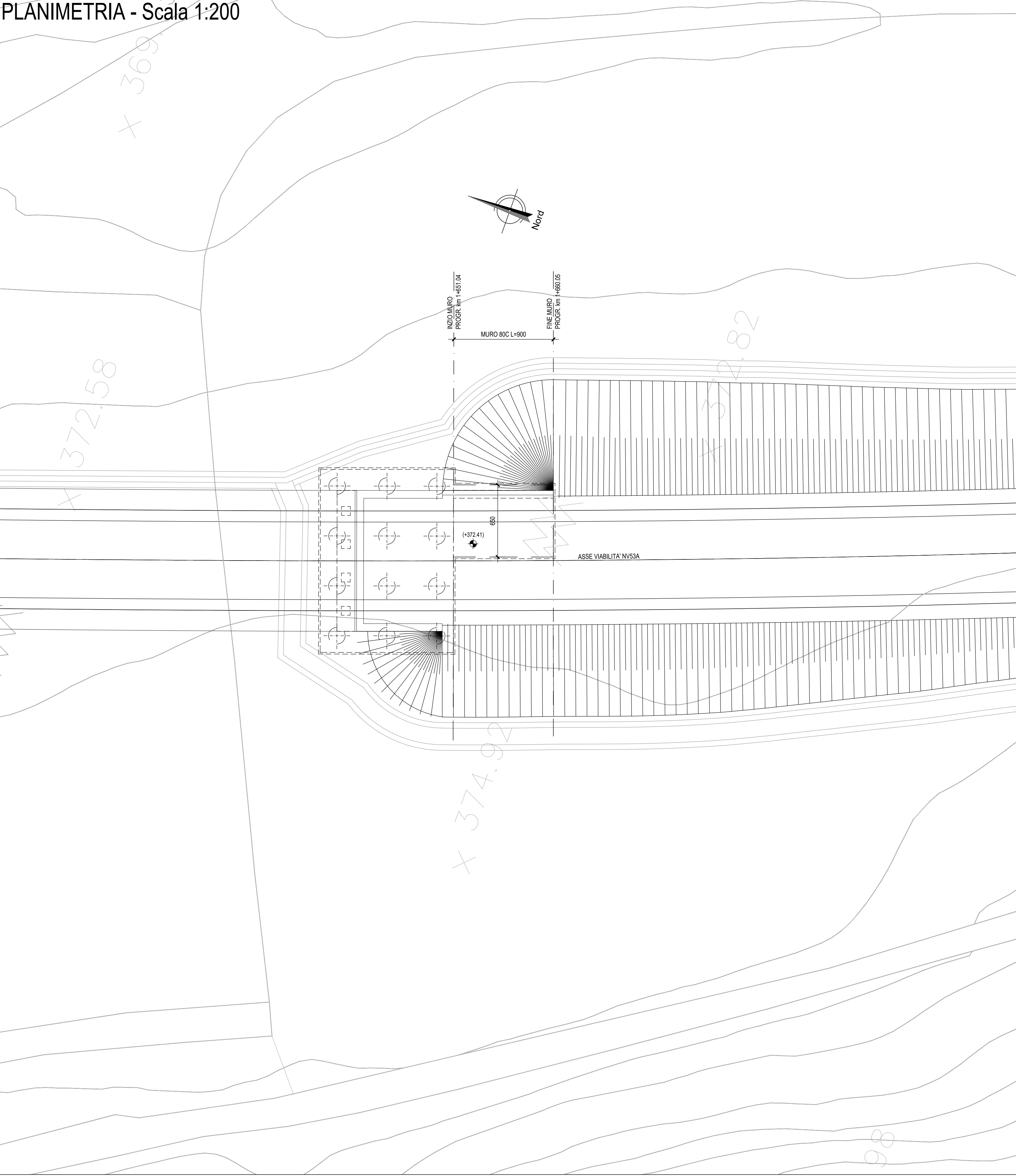
PLANIMETRIA - Scala 1:200
