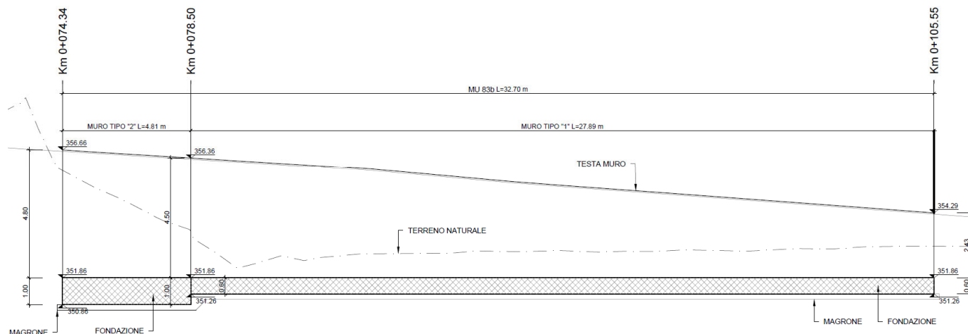
Figura 1-2 – NV58: Muro di sostegno MU83B - Prospetto.
