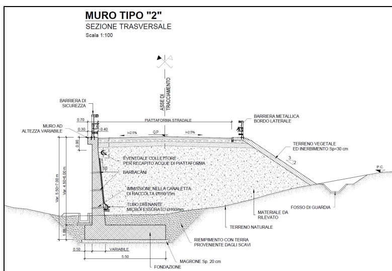
Figura 1-4 – NV58: Muro di sostegno MU83B – Sezione tipo 2.
