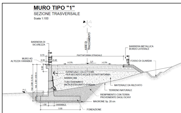
Figura 1-3 – NV58: Muro di sostegno MU83B – Sezione tipo 1.
