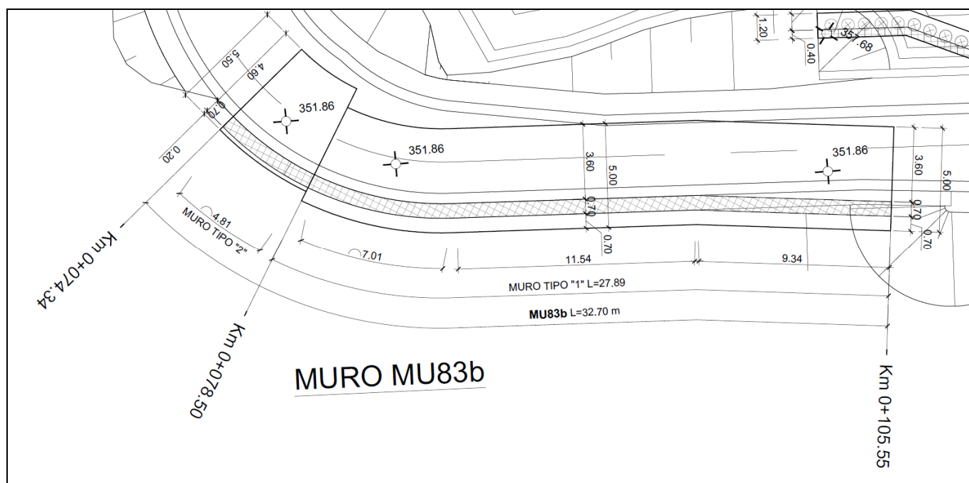
Figura 1-1 – NV58: Muro di sostegno MU83B - Pianta.
