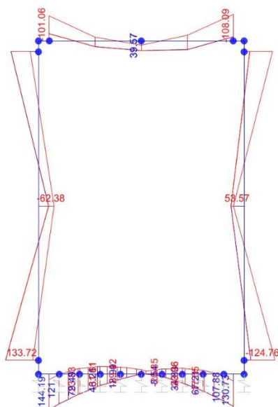
Momento Flettente
