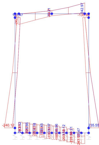
Taglio
