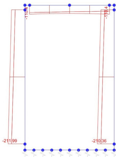
Sforzo normale
