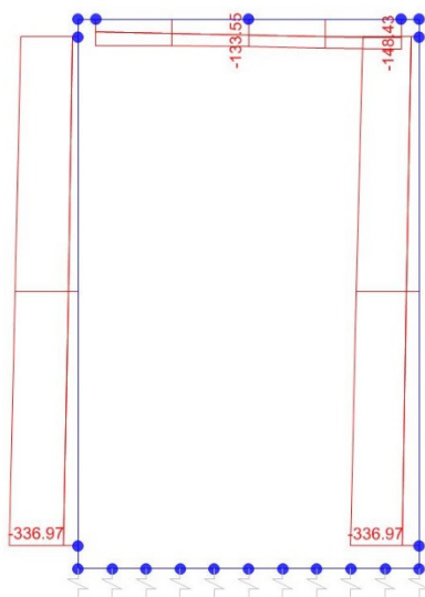
Sforzo normale
