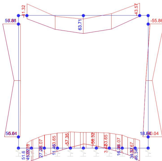
Momento Flettente
