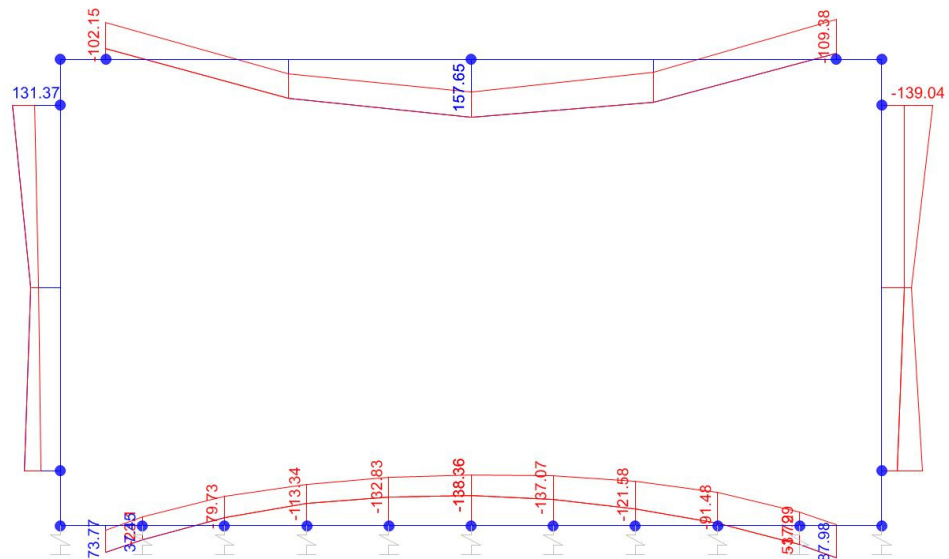
Momento Flettente
