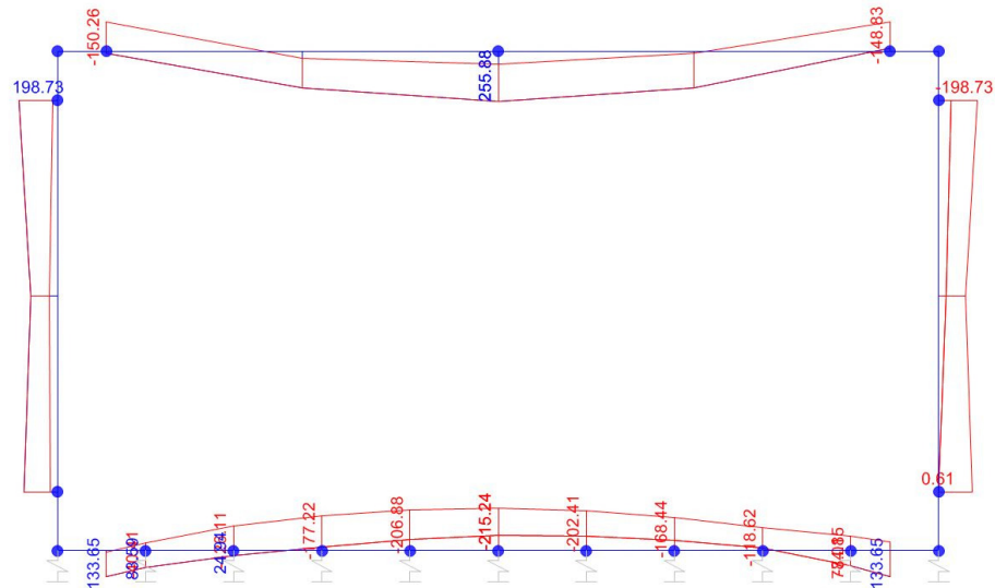
Momento Flettente
