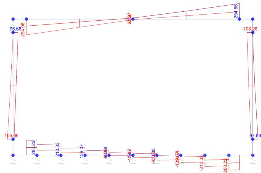
Taglio
