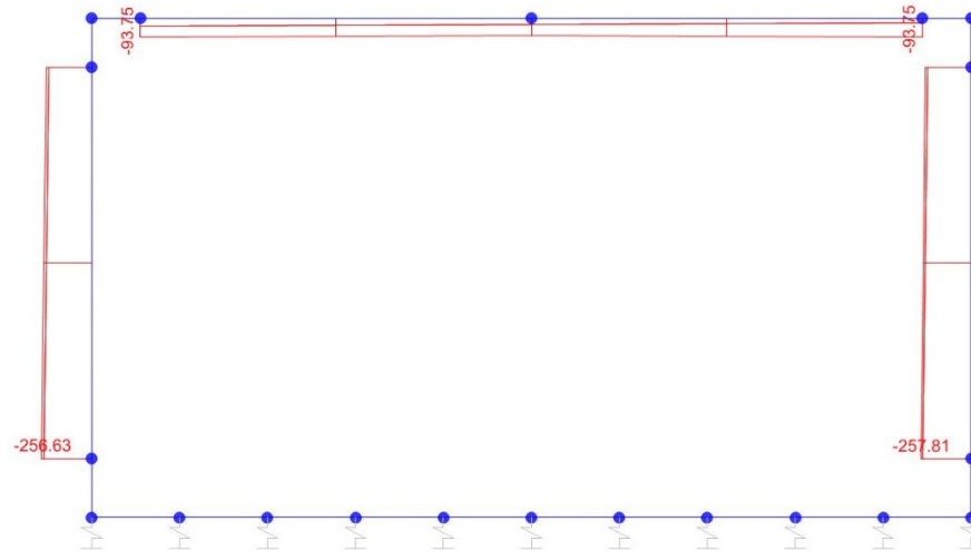
Sforzo normale
