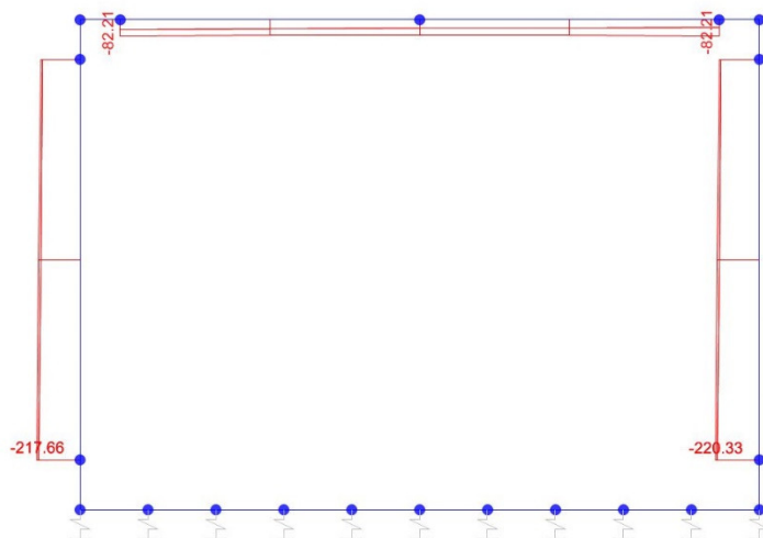
Sforzo normale
