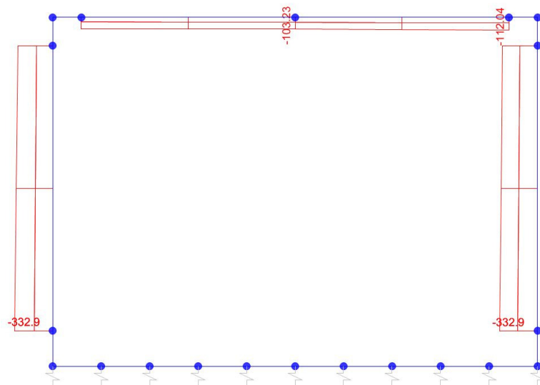
Sforzo normale
