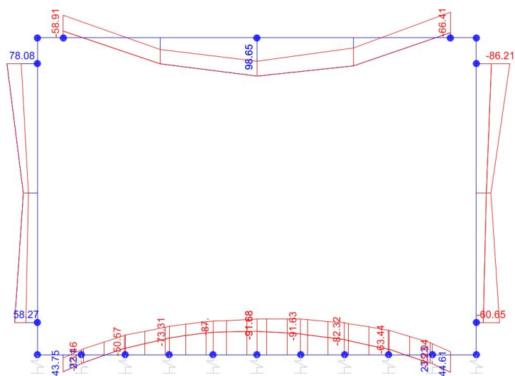
Momento Flettente
