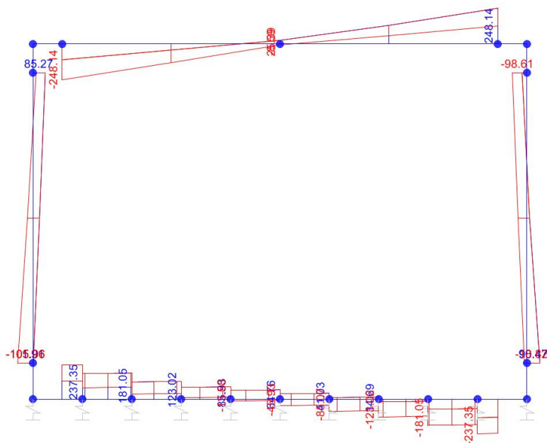
Taglio
