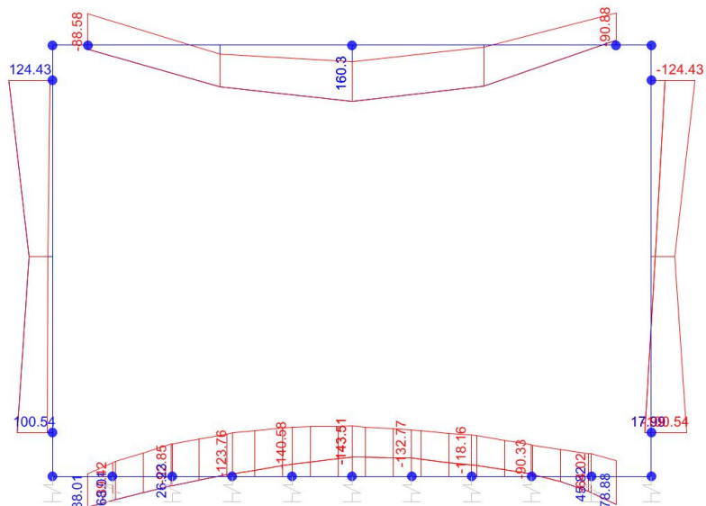
Momento Flettente
