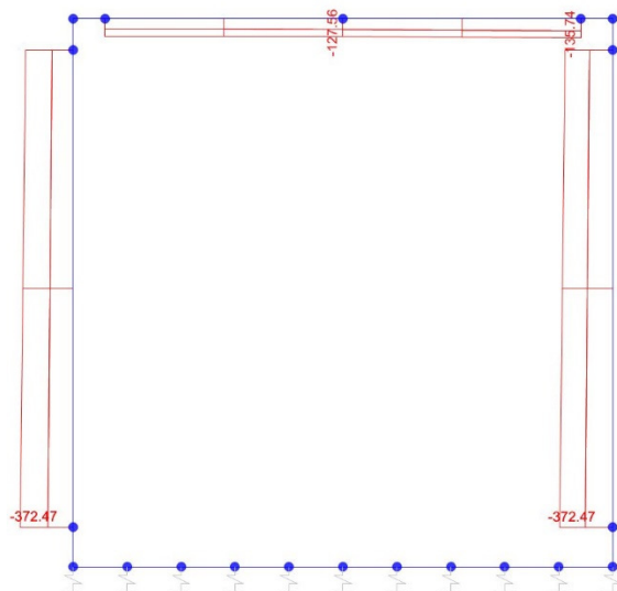
Sforzo normale
