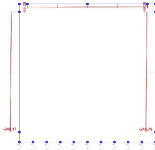
Sforzo normale
