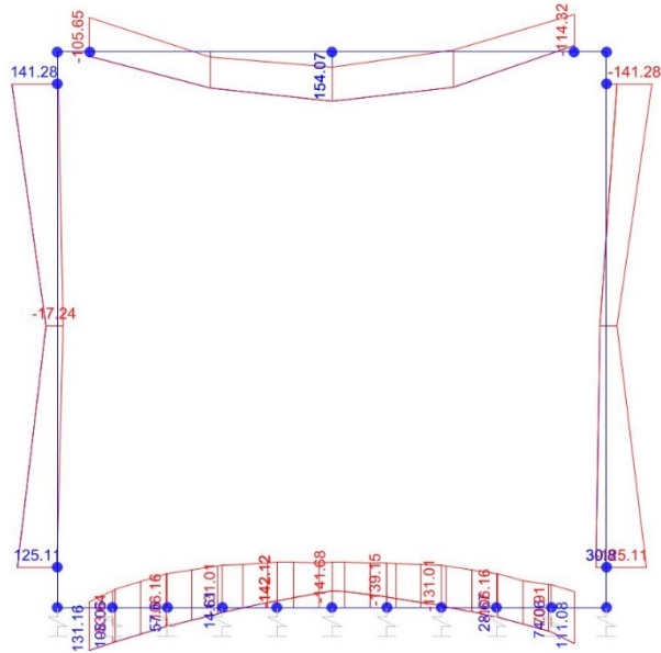
Momento Flettente
