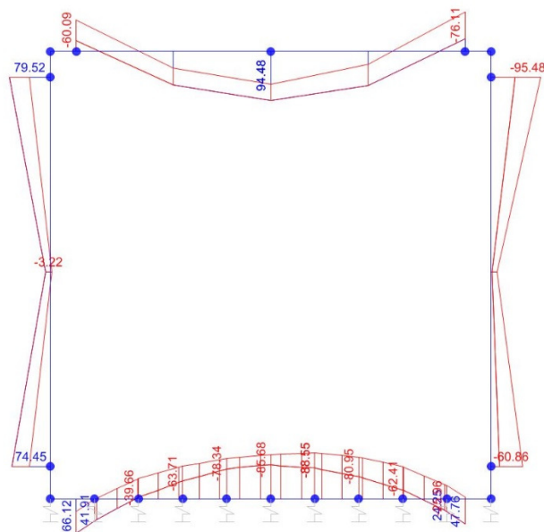
Momento Flettente
