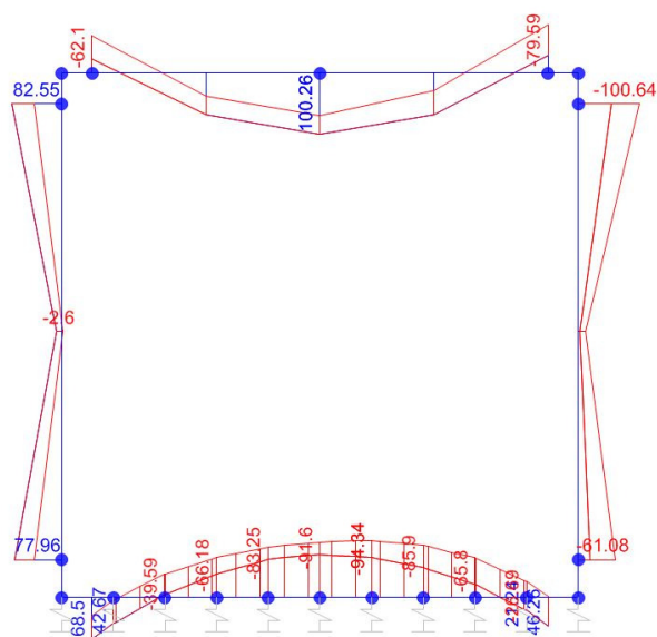
Momento Flettente
