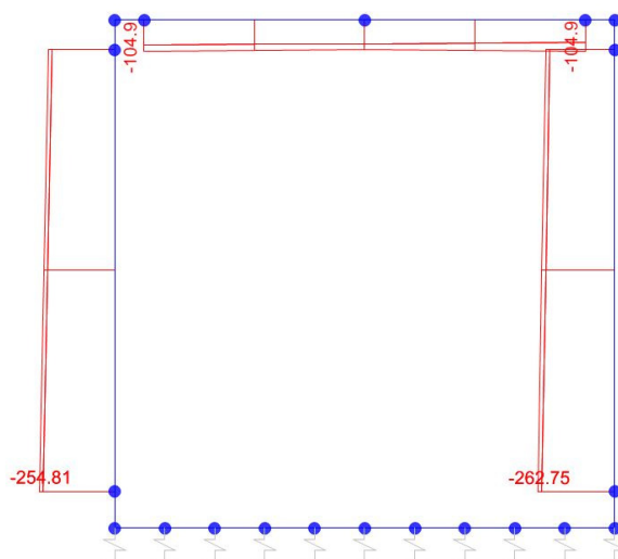
Sforzo normale
