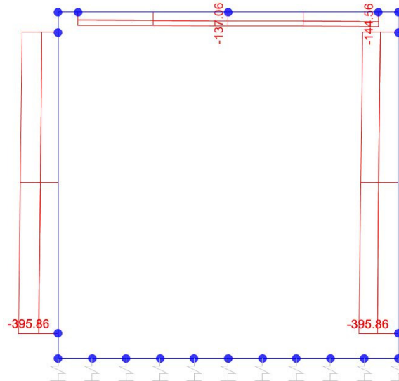
Sforzo normale
