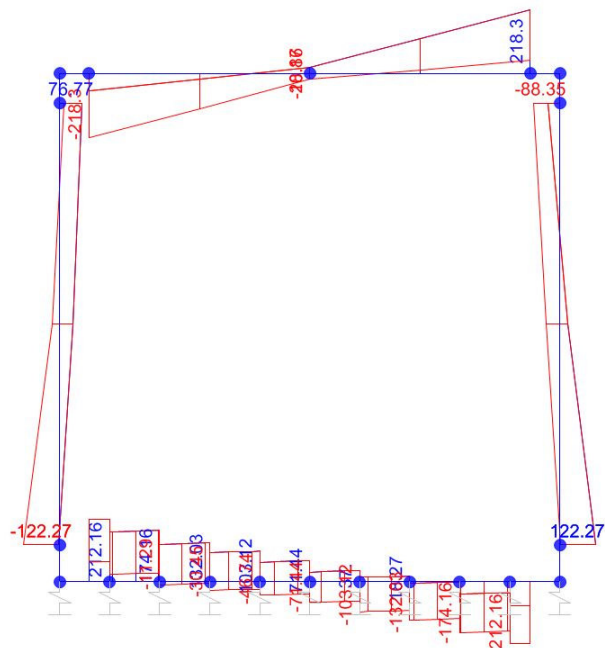
Taglio
