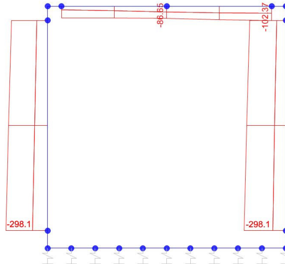
Sforzo normale
