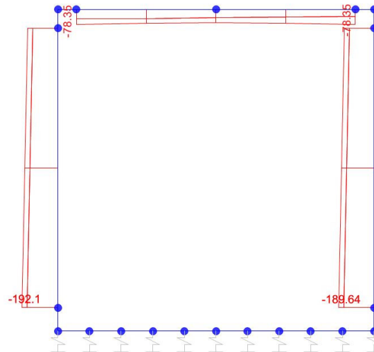
Sforzo normale
