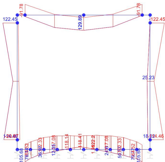
Momento Flettente
