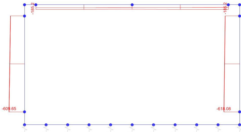
Sforzo normale
