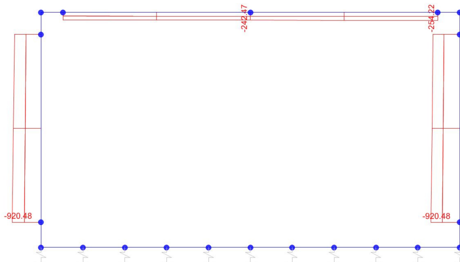
Sforzo normale
