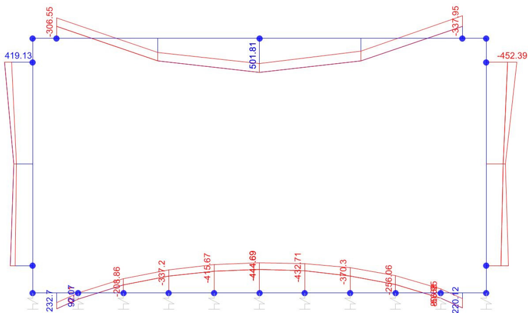
Momento Flettente
