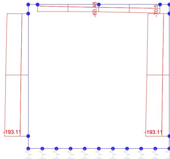
Sforzo normale
