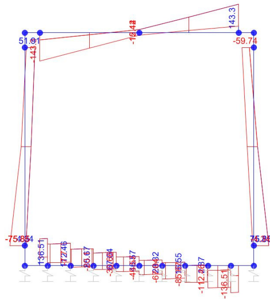
Taglio
