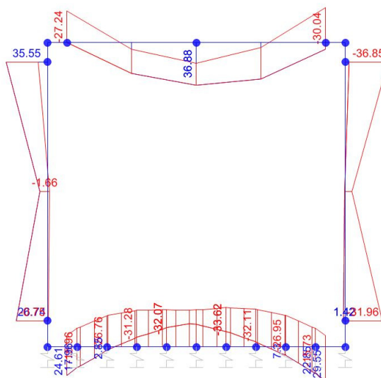
Momento Flettente
