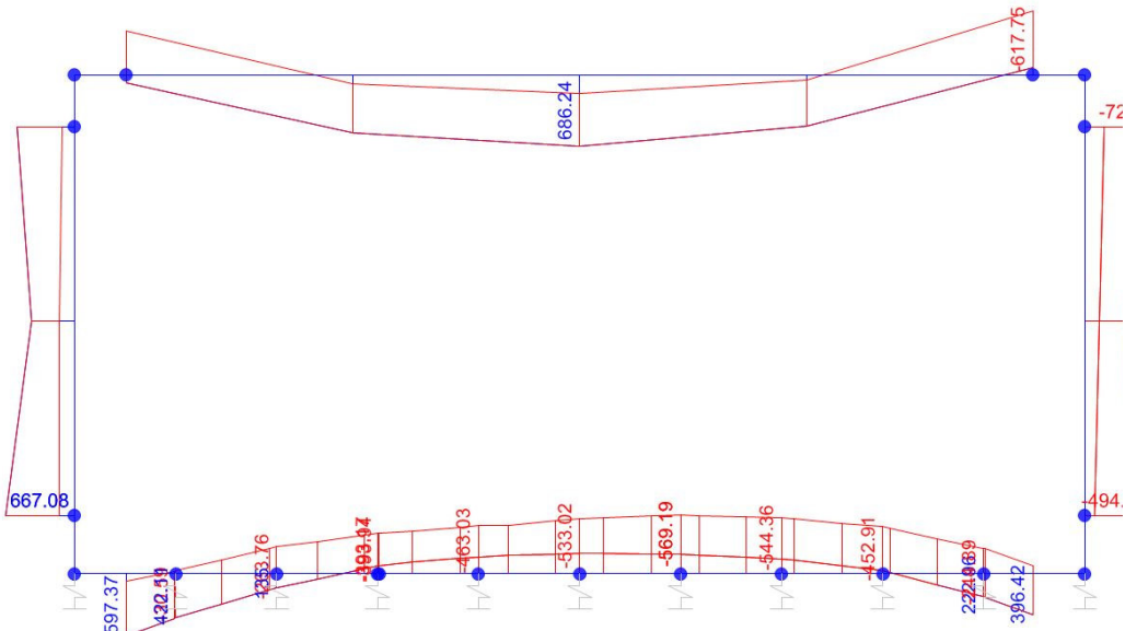
Momento Flettente
