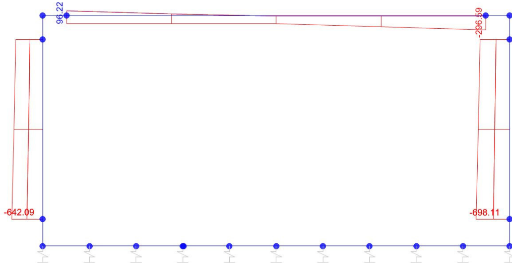
Sforzo normale
