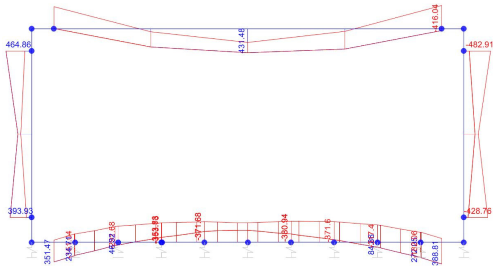
Momento Flettente
