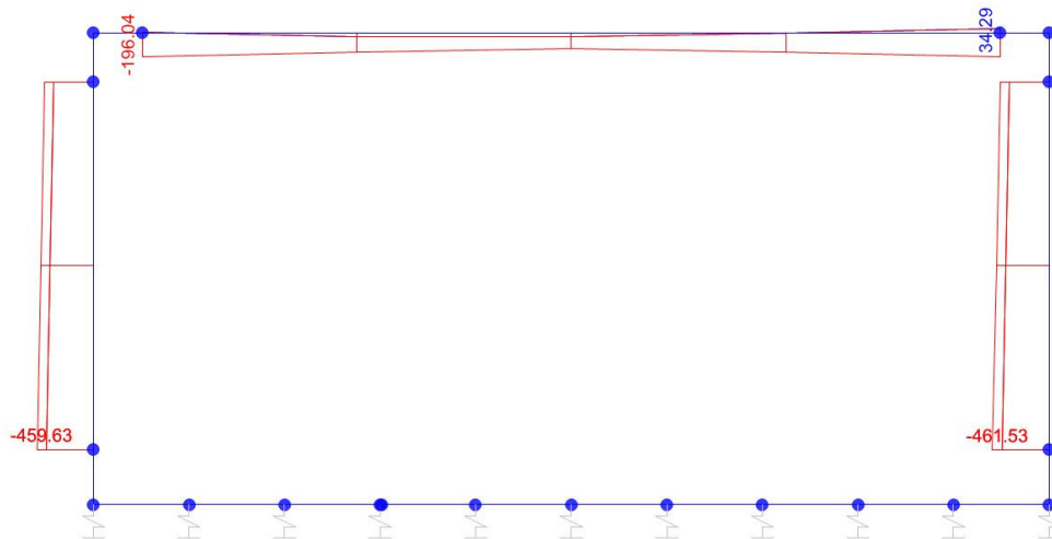
Sforzo normale
