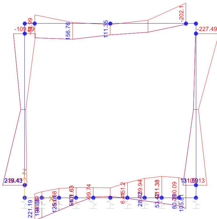
Momento Flettente
