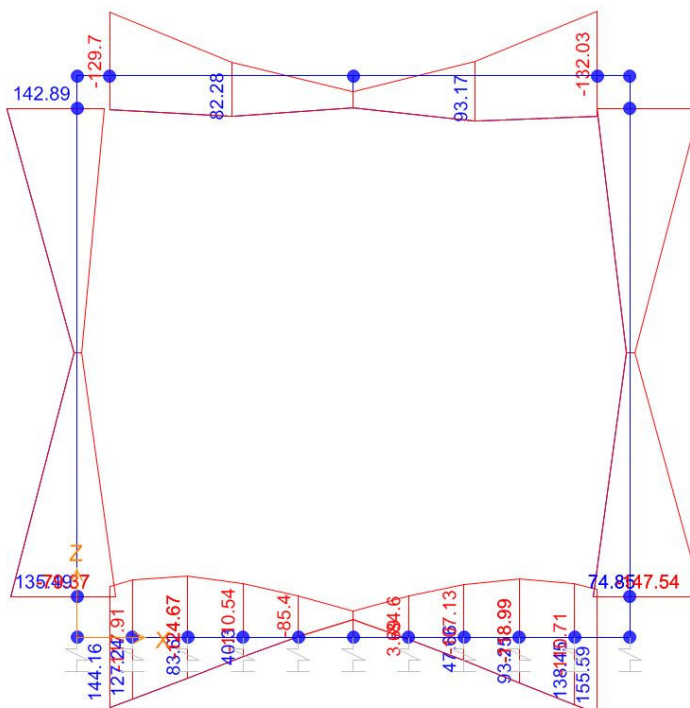
Momento Flettente
