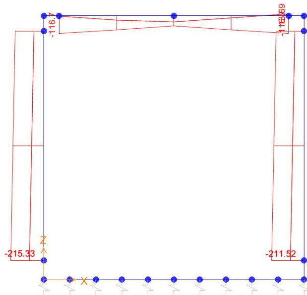
Sforzo normale
