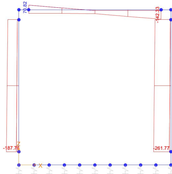
Sforzo normale
