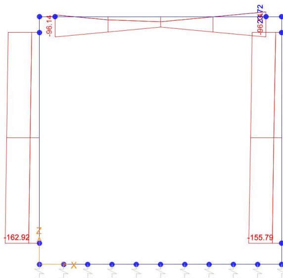
Sforzo normale
