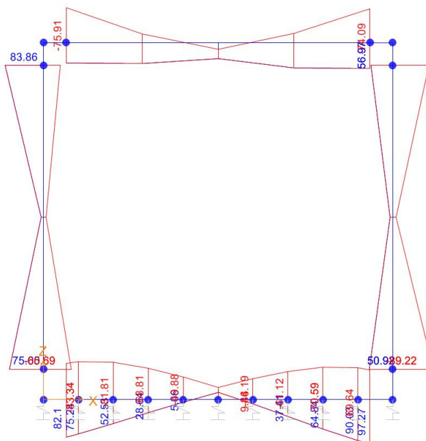
Momento Flettente
