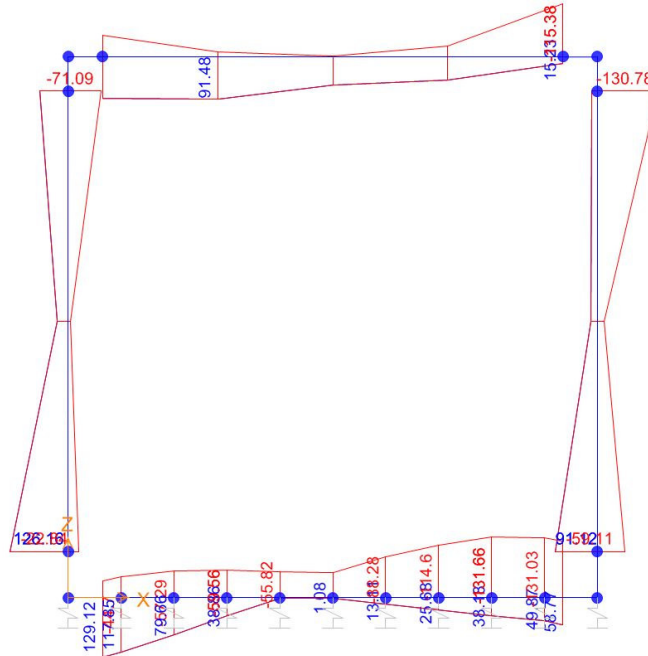
Momento Flettente
